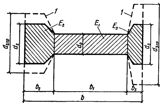
Рис. 14. Схема к определению размеров приведенного сечения контрфорса
