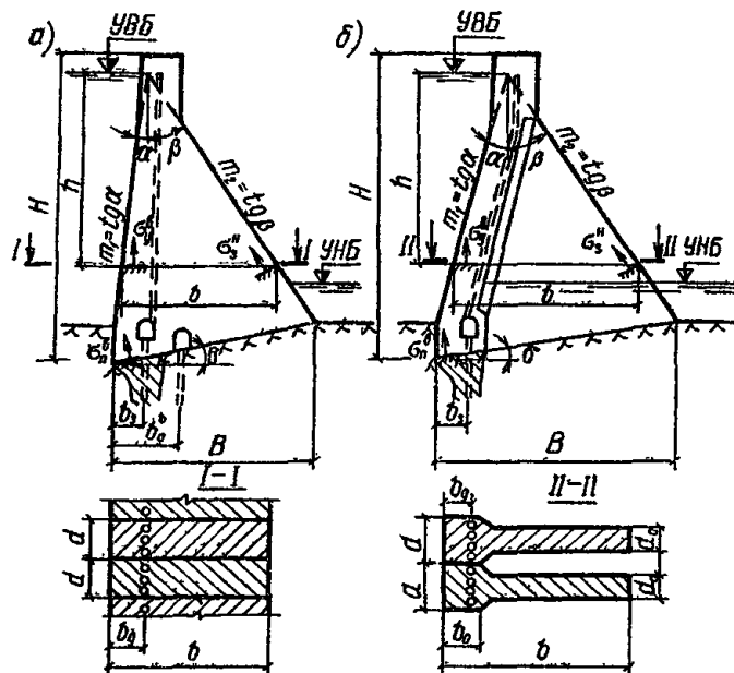
Рис. 11. Обозначения к расчету плотины на прочность
