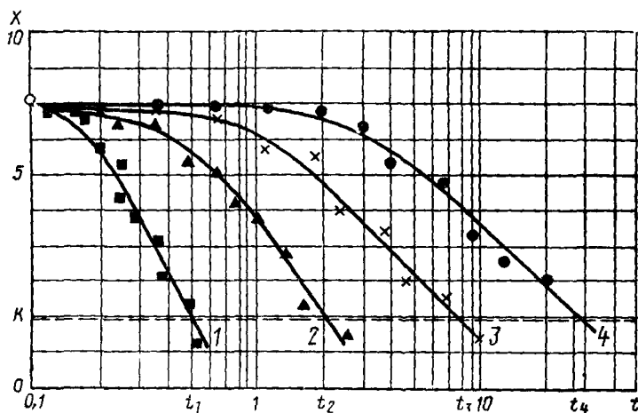
Способ определения среднего срока службы образцов t_1 — t_4 из кривых старения при непрерывном старении
