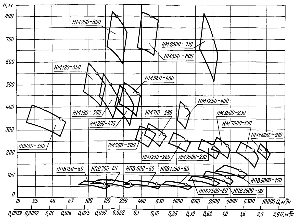
Поля Q-H
