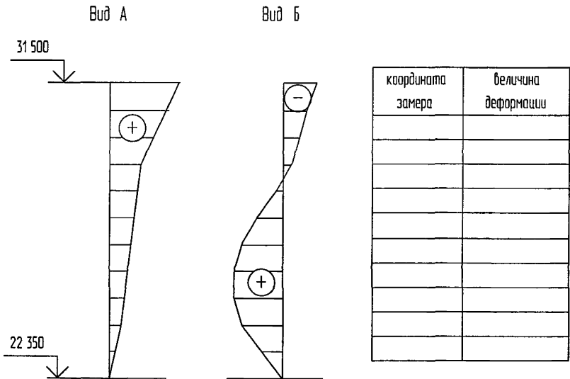
Этюра деформаций оси колонны К-1л
