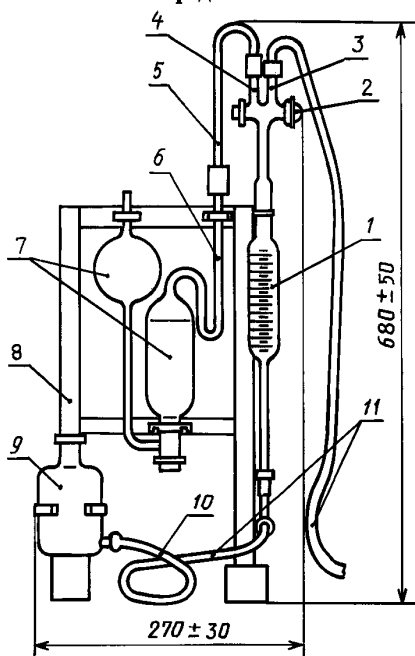
Измерительный аппарат для анализа кислорода АК-М1
