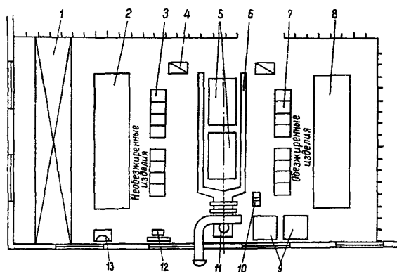
Черт. 19. Схематический план участка обезжиривания:
