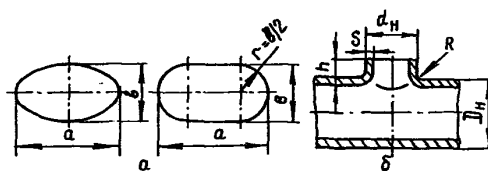
Черт. 4. Форма отверстия (а) для ответвлений в трубах (б)
