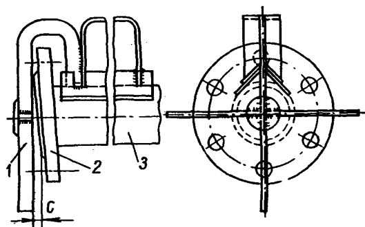
Черт. 13. Контроль отклонения от перпендикулярности уплотнительной поверхности фланца:
