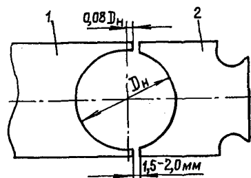
Черт. 7. Зазор между ползуном и ги- бочным диском:
