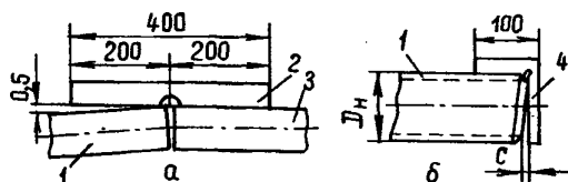
Черт. 12. Контроль прямолинейности (а) и неперпендикулярности торцов (б) собираемых элементов:
