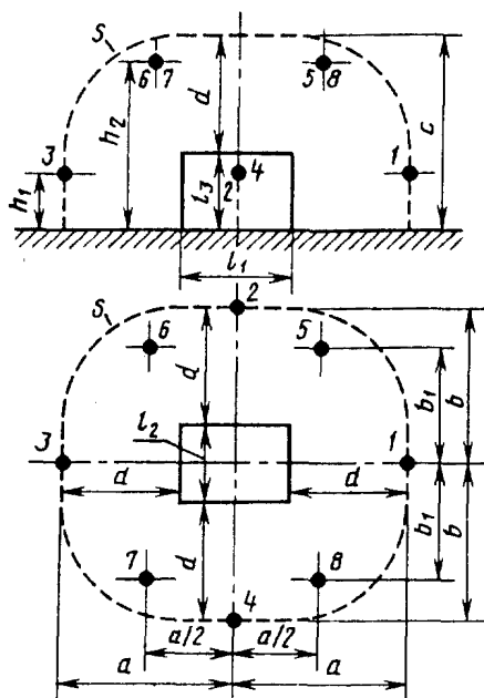
S — измерительная поверхность; 1 — 8 — точки измерения; l_1, l_2, l_3 — размеры огибающего источника шума параллелепипеда; d — измерительное расстояние; a, b, c — характеристические размеры измерительной поверхности
