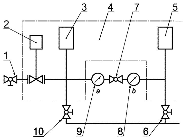
1, 6, 7, 10 — краны; 2 — испытываемый образец; 3, 5 — воздушный резервуар объемом 1 дм 3 ; 4 — отсек постоянной температуры; 8, 9 — манометры
