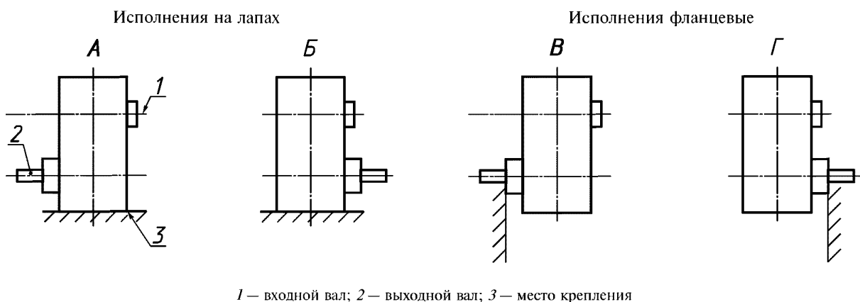
Рисунок А.1 — Варианты сборки
