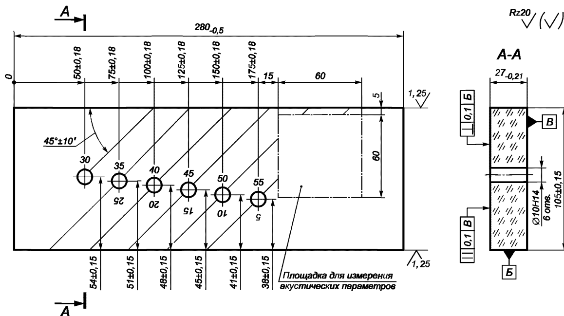
Рисунок 2 — Стандартный образец СО-1Р
