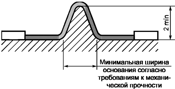
Рисунок Е.1 — Размеры ребер
