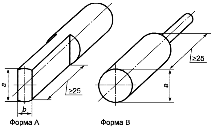
Рисунок 5 — Щупы (см. 9.2.4.5)
