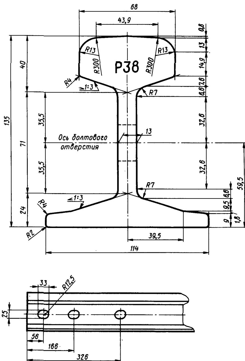
Черт. 38. Рельс типа Р38 (II-а) по ГОСТ 3542—47
