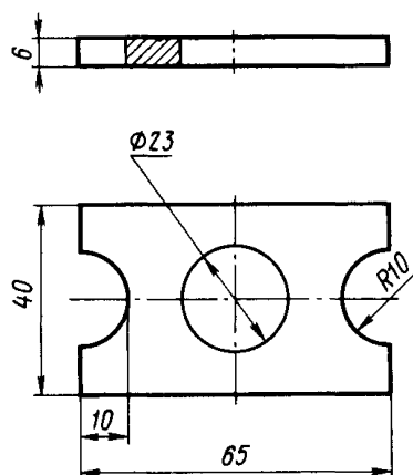
Черт. 85. Скоба для изолирующей втулки КБ
