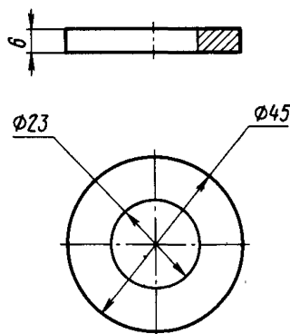
Черт. 84. Шайба черная 22
