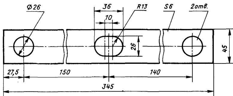
Черт. 154. Планка стопорная СИ-50-2
