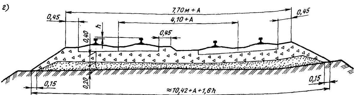
Черт. 6. Поперечные профили балластной призмы из щебня на песчаной подушке для особо тяжелого типа верхнего строения пути на двухпутных участках: а, б — соответственно в прямых и кривых на деревянных шпалах; в, г — то же на железобетонных шпалах; А — уширение междупутья в кривых; h — возвышение наружного рельса; 1 — щебень; 2 — песок
