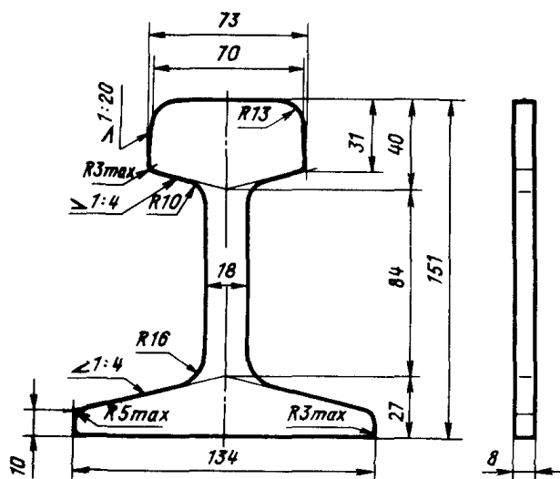
Черт. 156. Прокладка стыковая ПС-50
