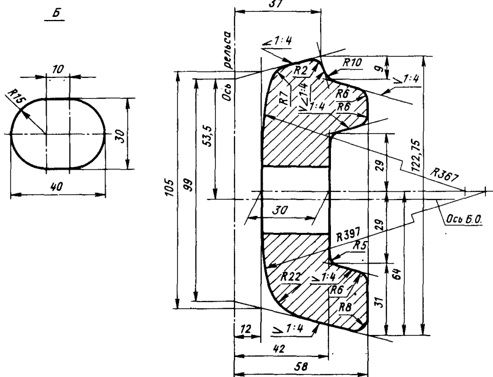
Черт. 138. Накладка специальная для изолирующих стыков типа Р65
