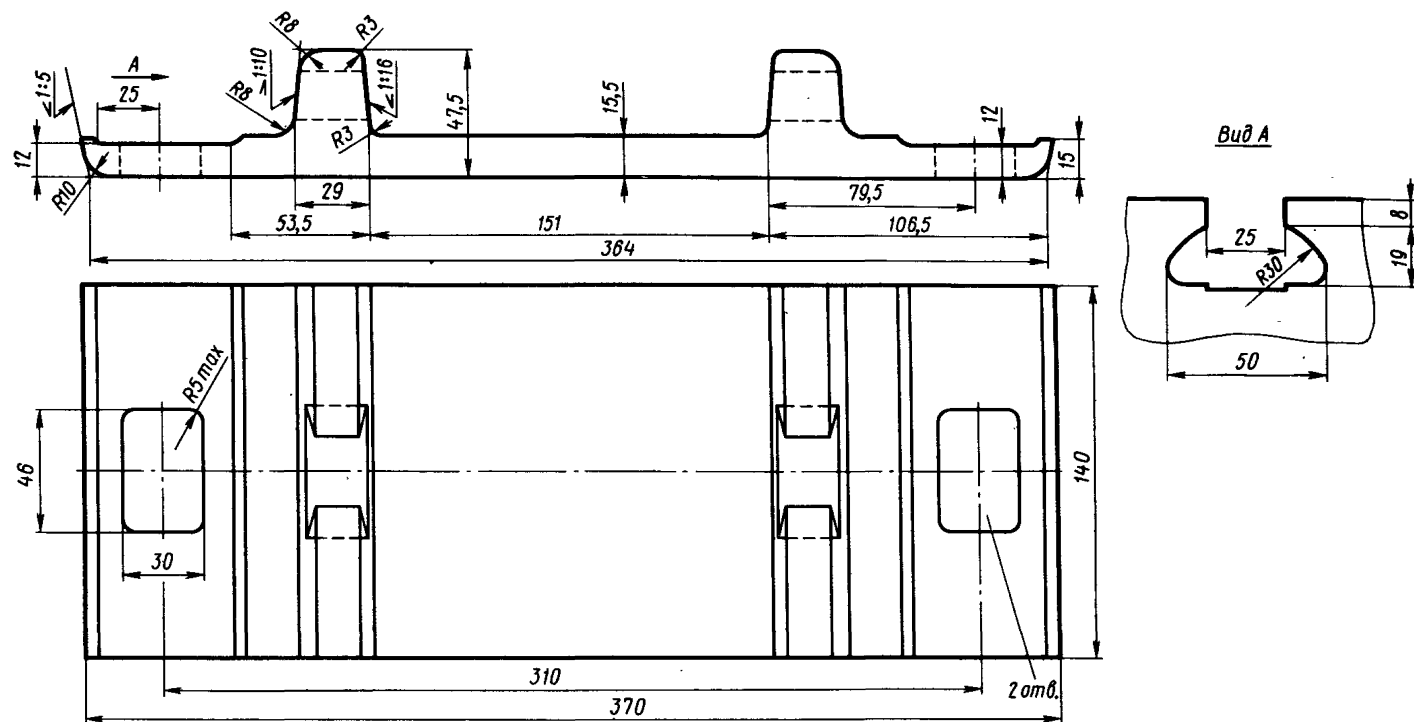
Черт. 78. Подкладка раздельного крепления KB65 по ГОСТ 16279—78
