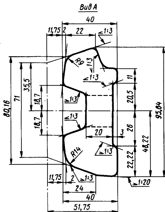
Черт. 50. Накладка двухголовая к рельсам типа Р43 по ГОСТ 19127—73: а — шестидырная; б — четырехдырная
