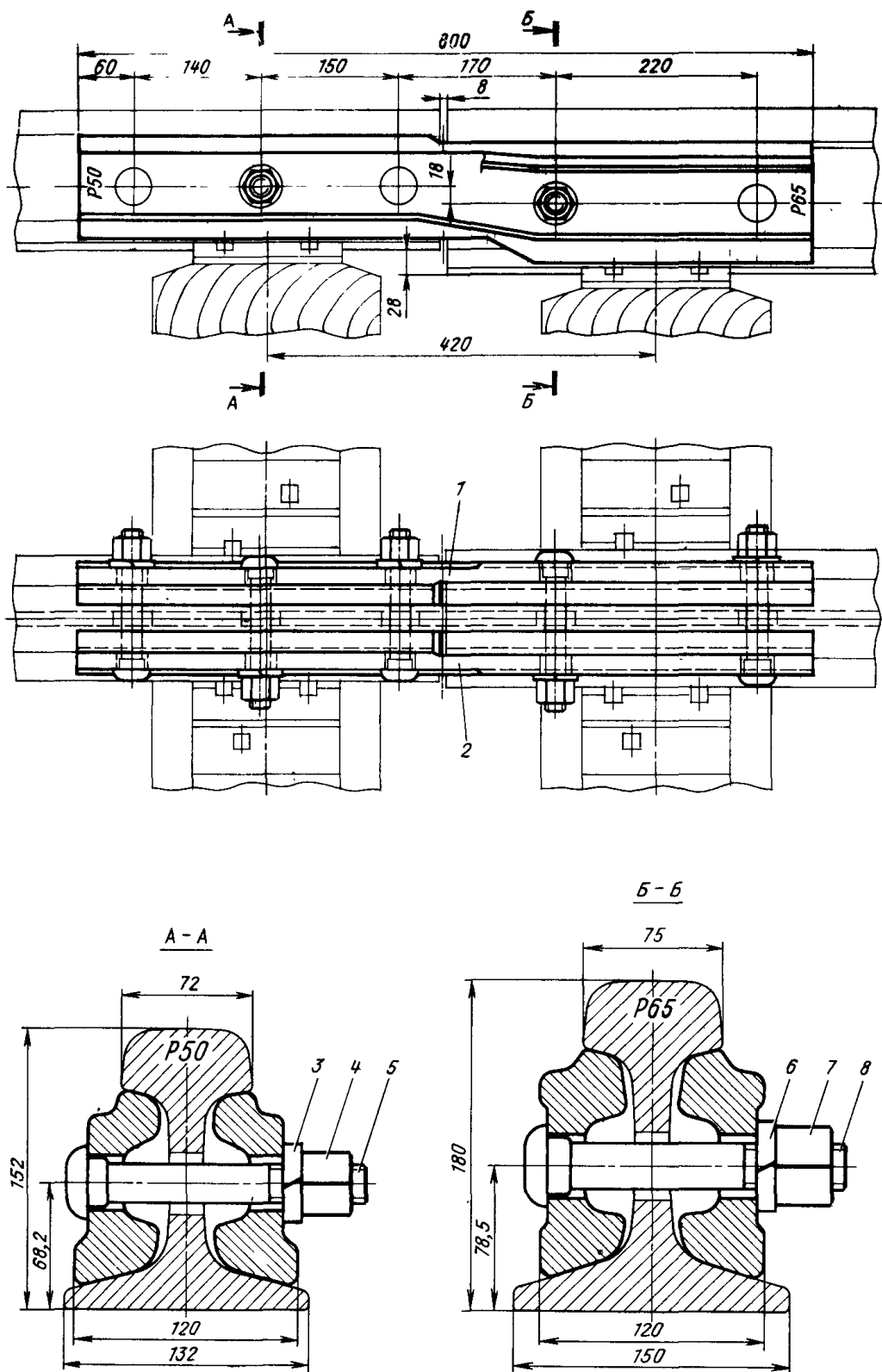
Черт. 118. Переходный стык рельсов P65 — P50
