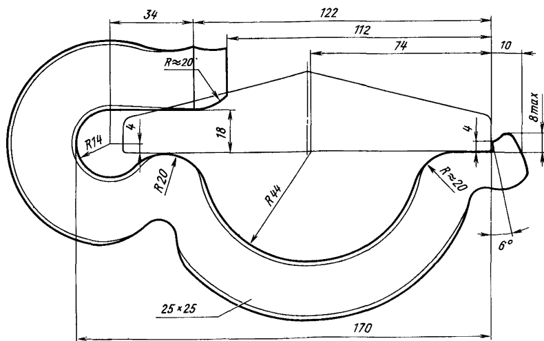
Черт. 71. Противоугоны пружинные П75 по ТУ 14-4-1438—87 к рельсам типа Р75
