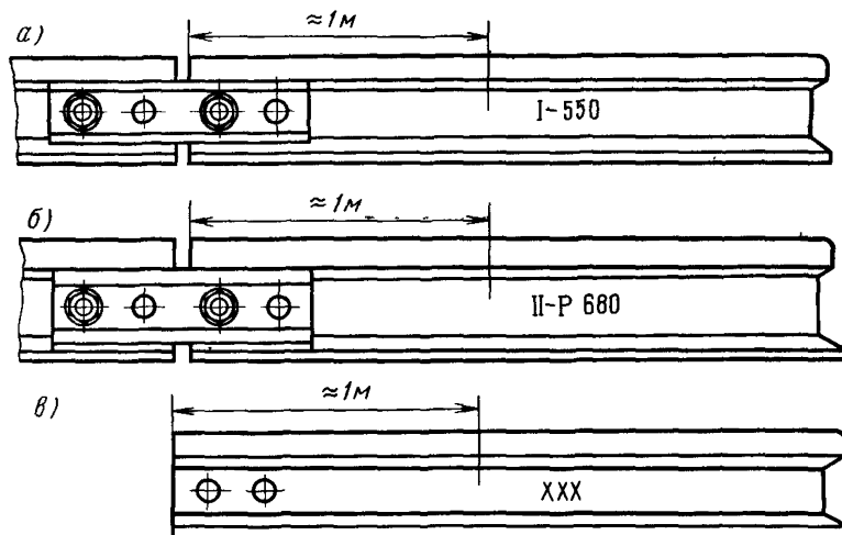
Черт. 42. Пример маркировки старогодных рельсов (светлой краской):
