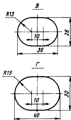
Черт. 119. Накладка переходная P65 — P50 (правая)
