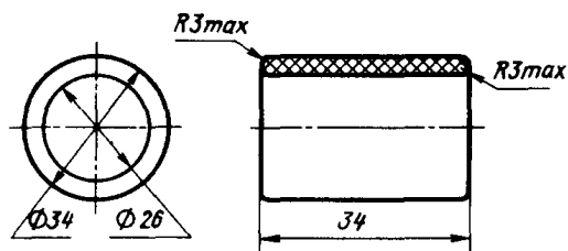
Черт. 157. Втулка В-24
