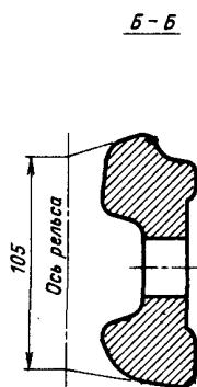
Черт. 119. Накладка переходная P65 — P50 (правая)
