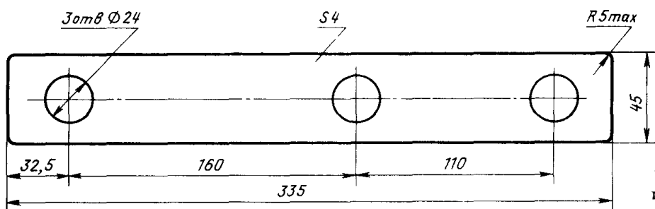
Черт. 161. Прокладка боковая составная ПБС-43
