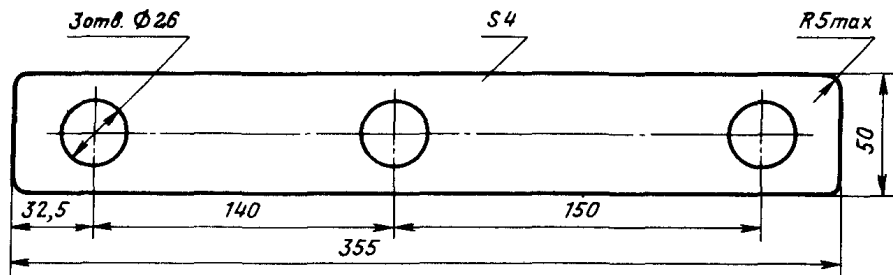
Черт. 155. Планка под болты ПТБ-50
