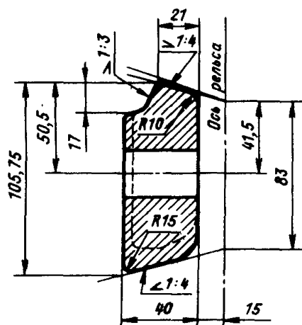
Черт. 133. Планка стопорная С-43-1
