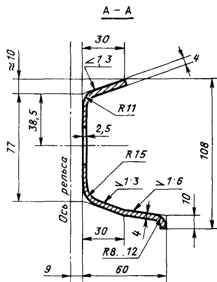
Черт. 161. Прокладка боковая составная ПБС-43
