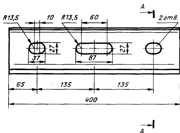
Черт. 161. Прокладка боковая составная ПБС-43
