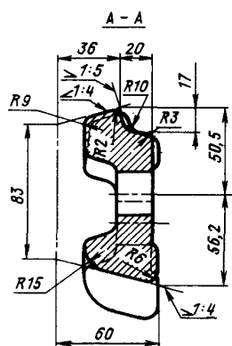
Черт. 119. Накладка переходная P65 — P50 (правая)
