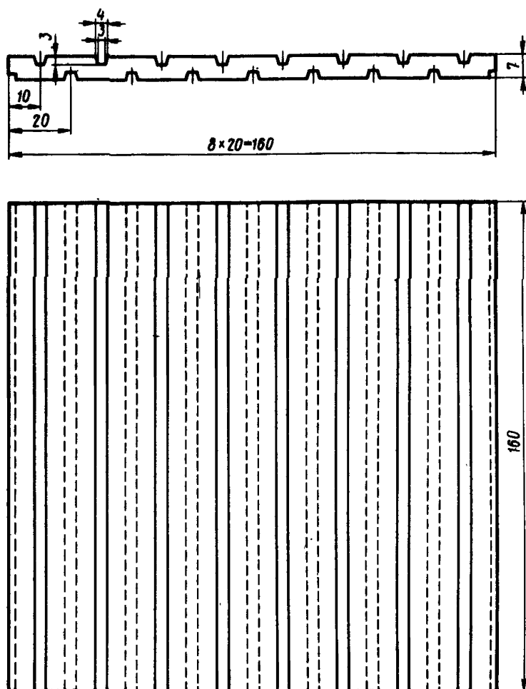
Черт. 105. Прокладка амортизирующая
