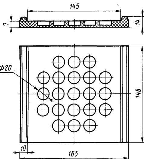
Черт. 83. Прокладка под подошву рельсов Р65
