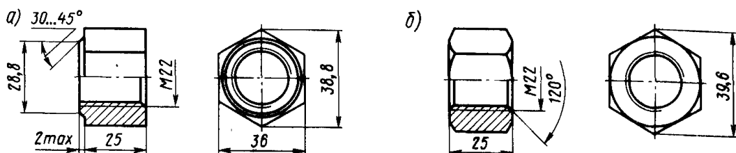
Черт. 57. Гайка M22 по ГОСТ 11532—76 к болтам для рельсов типов Р43, Р38, I-а и Р33: а — с одной фаской; б — с двумя фасками
