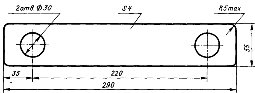
Черт. 145. Планка под болты ППБ-65
