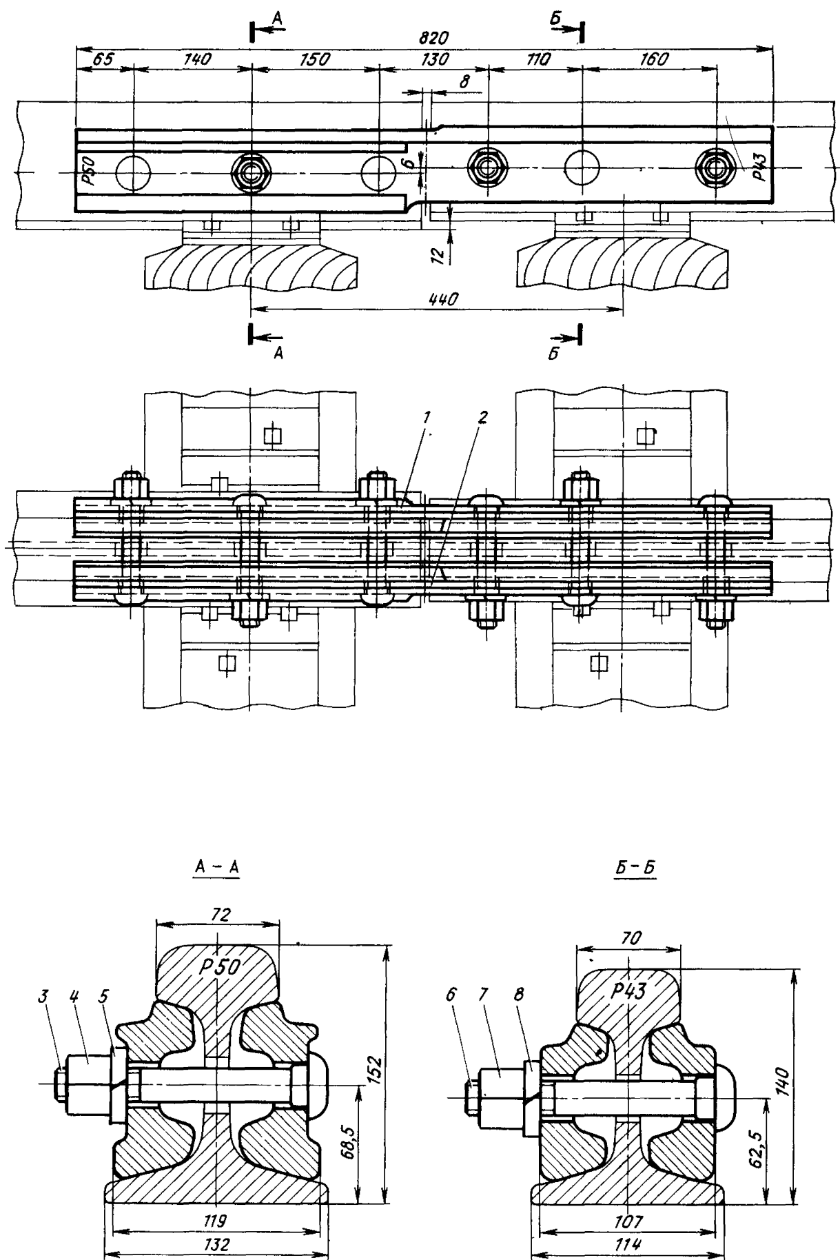
Черт. 127. Переходный стык рельсов Р50 — Р43
