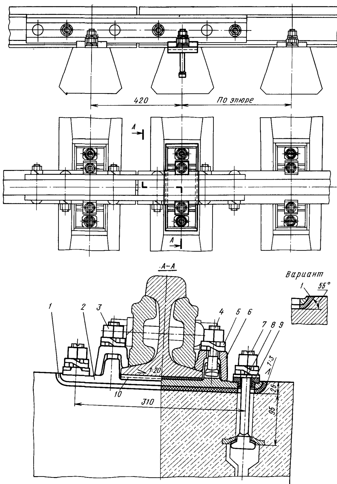
Черт. 77. Рельсовое крепление KB65 на железобетонных шпалах с рельсами типов P65 и P75
