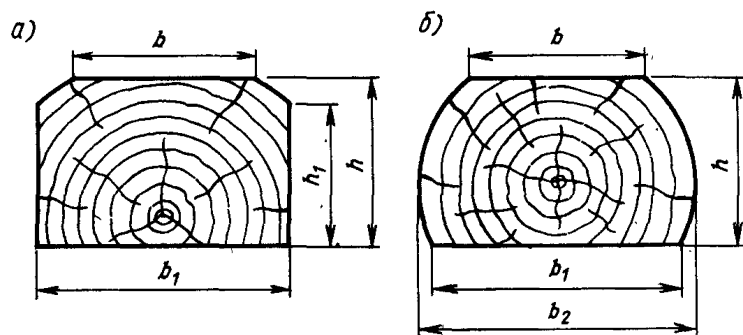
Черт. 15. Поперечные сечения деревянных брусьев для стре- лочных переводов по ГОСТ 8816—70: a — обрезных; b — необрезных
