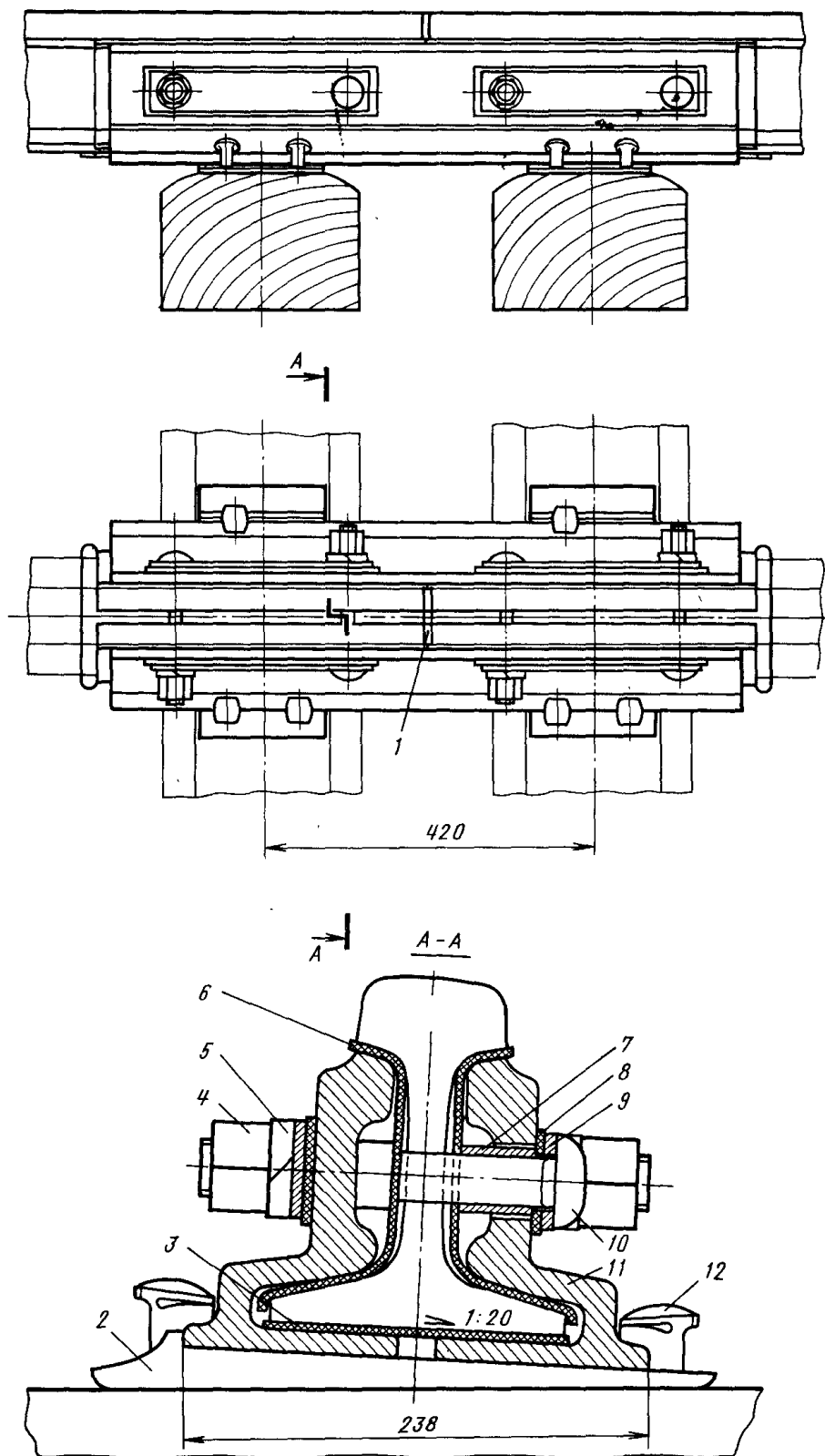
Черт. 139. Изолирующий стык рельсов типа Р65 с объёмлющими накладками на деревянных шпалах
