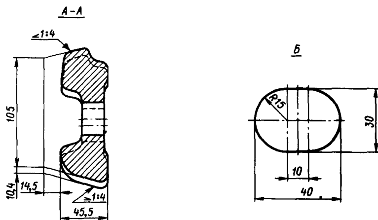
Черт. 116. Накладка переходная Р75 — Р65 (правая)
