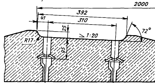
Черт. 18. Шпала железобетонная типа ШС-1 по ГОСТ 10629—78: 1 — арматура; 2 — закладная шайба
