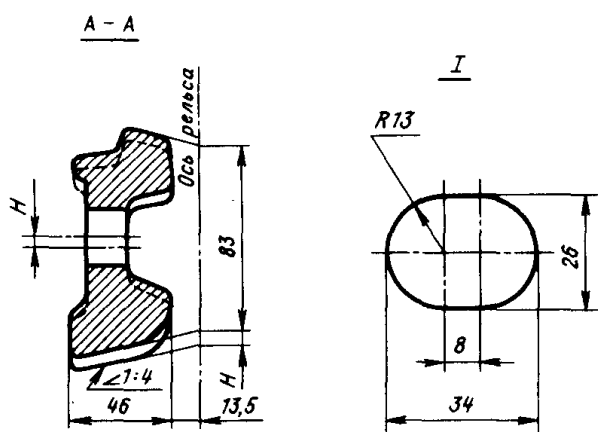
Черт. 126. Накладка переходная Р50 — Р50 (левая) (Величина перегиба Н должна соответствовать вертикальному износу головки рельса)
