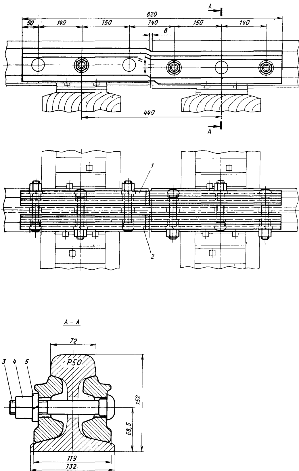
Черт. 124. Переходный стык рельсов P50 — P50
