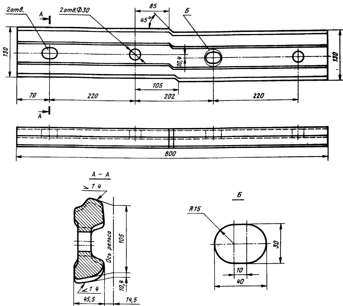
Черт. 117. Накладка переходная Р75 — Р65 (левая)
