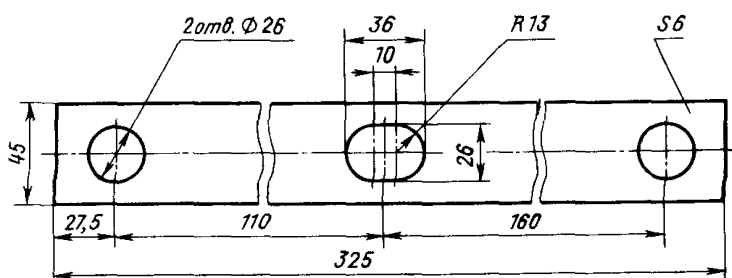
Черт. 134. Планка стопорная С-43-2
