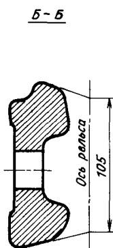
Черт. 120. Накладка переходная P65 — P50 (левая)
