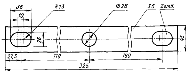
Черт. 132. Накладка переходная P50 — P43 из полосы (левая)
