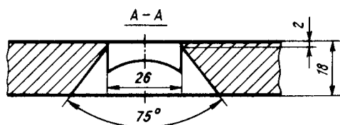
Черт. 172. Подкладка для рельсов типа Р50
