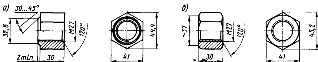
Черт. 53. Гайка M27 по ГОСТ 11532—76 к болтам для рельсов типов Р65 и Р75: а — с одной фаской; б — с двумя фасками
