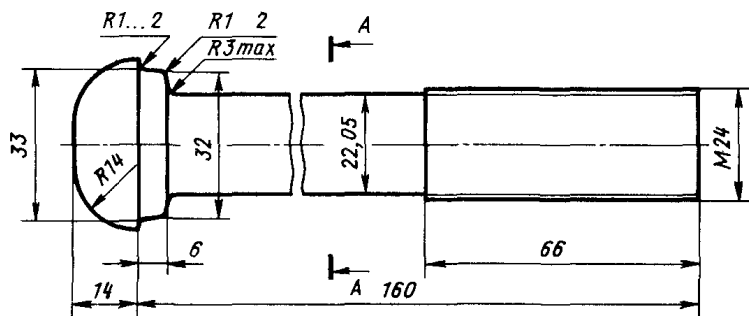
Черт. 158. Болт 2М24×160 ГОСТ 11530—76
