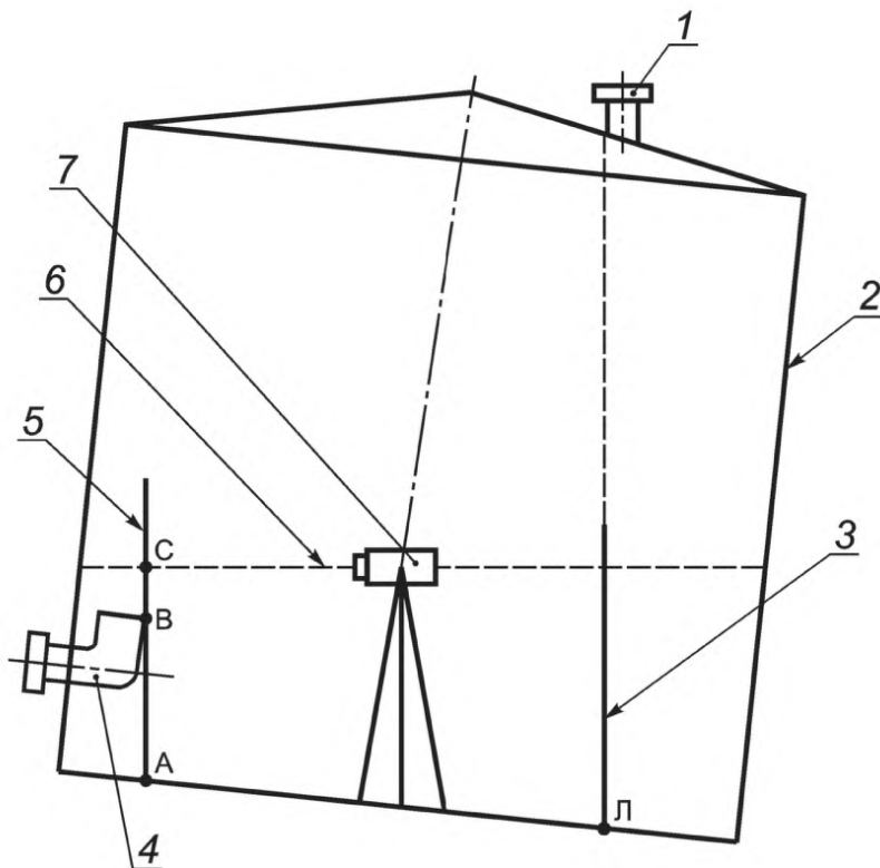
1 — измерительный люк; 2 — резервуар; 3 — рейка, установленная в точке Л; 4 — приемно-раздаточное устройство (ПРУ); 5 — рейка, установленная в точке А; 6 — горизонт нивелира; 7 — нивелир; А, Л — точки установки рейки; В, С — точки отсчета по рейке
