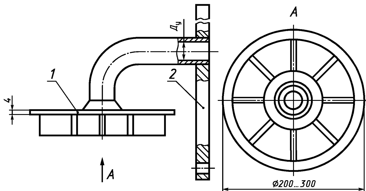
1 — воронкогаситель; 2 — крышка люка-лаза
