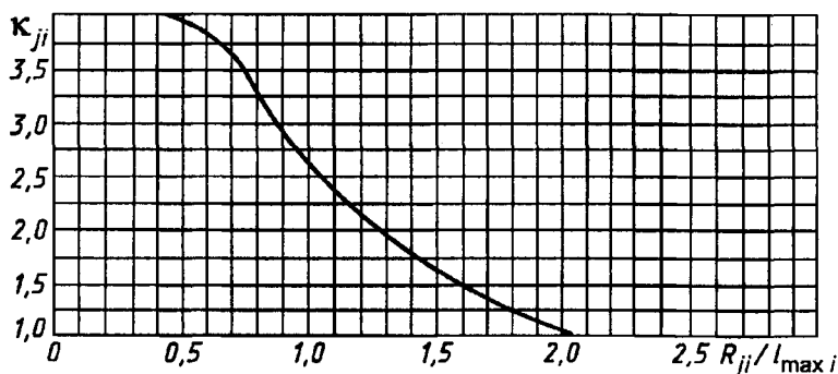
Рисунок Б.1 — График для определения параметра k_{ji} , учитывающего влияние ближнего звукового поля на значения уровней шума, создаваемого i -й машиной на j -м рабочем месте
