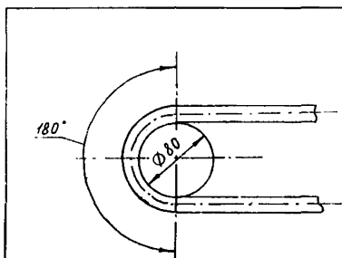
Рисунок 5. Схема определения работоспособности воздуховодного шланга
