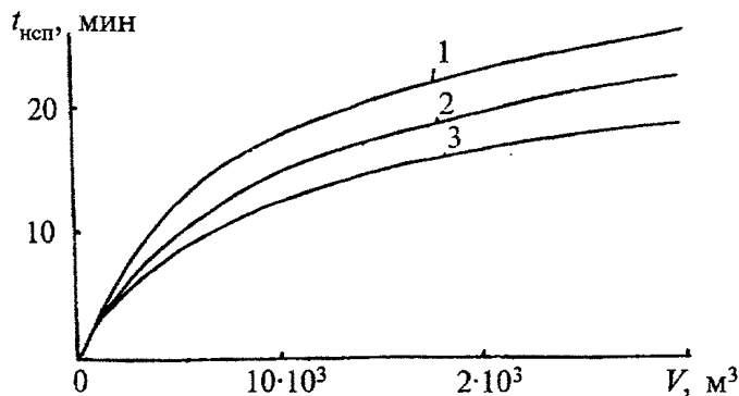
Рис. 5. Зависимость минимальной продолжительности начальной стадии пожара t_{\text{нсп}} от объема V и высоты H помещения
