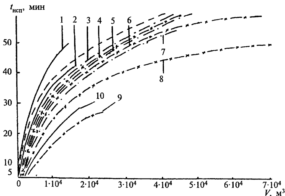
Рис. 4. Зависимость минимальной продолжительности начальной стадии пожара t_{\text{нсп}} от объема V , высоты H помещения и количества пожарной нагрузки g
