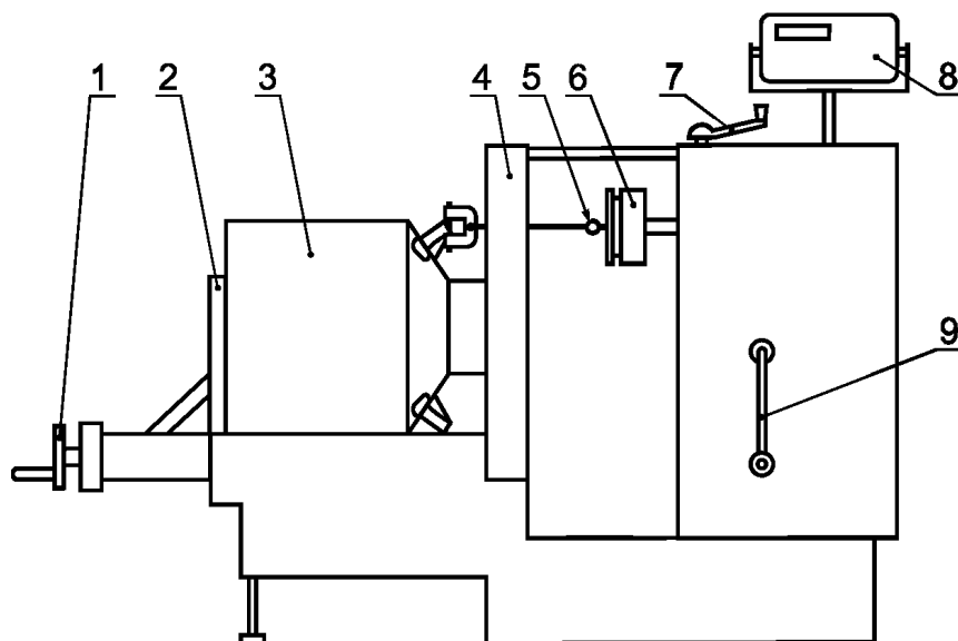
1 — устройство прижима тары; 2 — подвижный упор; 3 — испытываемая тара; 4 — неподвижный упор; 5 — серьга; 6 — датчик усилия; 7 — рукоятка привода гидронасоса; 8 — цифровой вольтметр; 9 — рукоятка подъема гидроцилиндра
