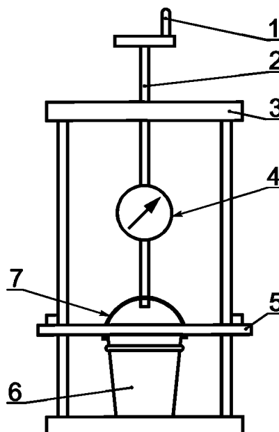
Рисунок Б.1 — Схема универсального устройства для испытания элементов тары на прочность с контролем измерения усилия по динамометру
