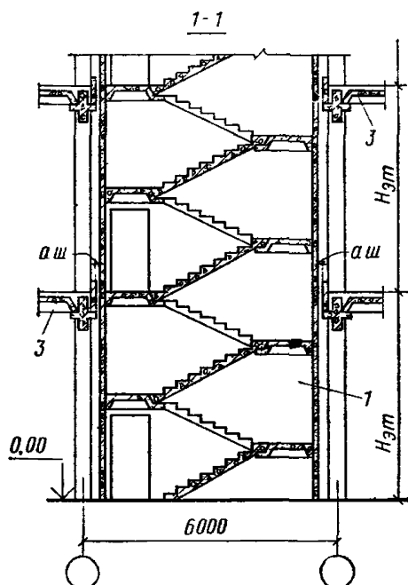
Рис. 93. Схема встроенной отдельно стоящей лестничной клетки
