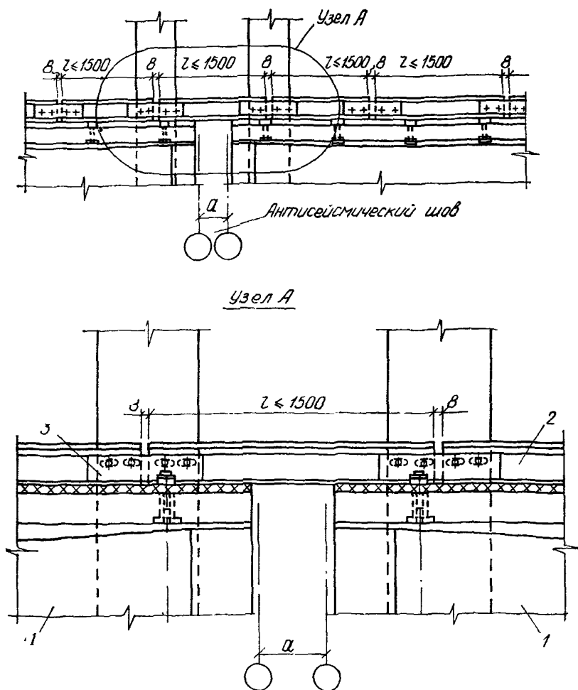
Рис. 11. Стык крановых рельсов вблизи антисейсмического шва
