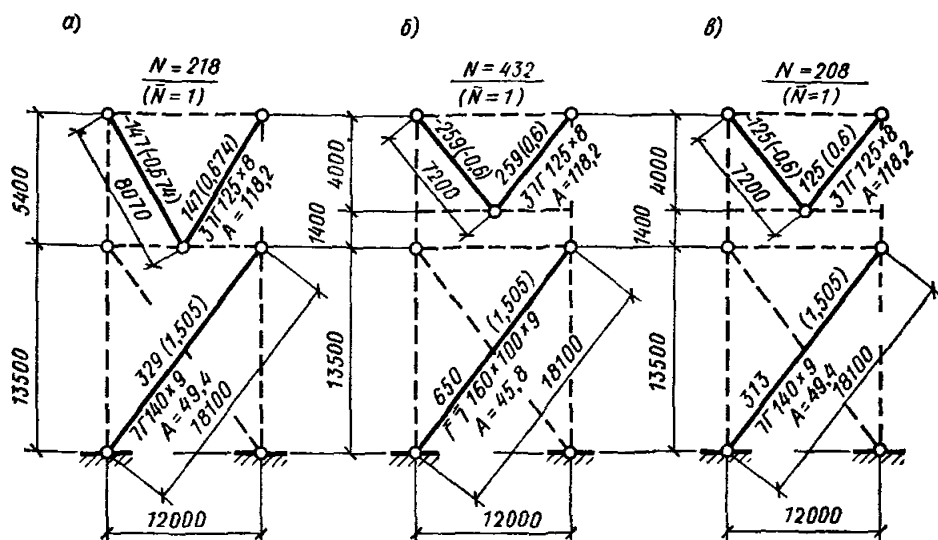
Рис. 133. Расчетные геометрические схемы связей по колоннам
