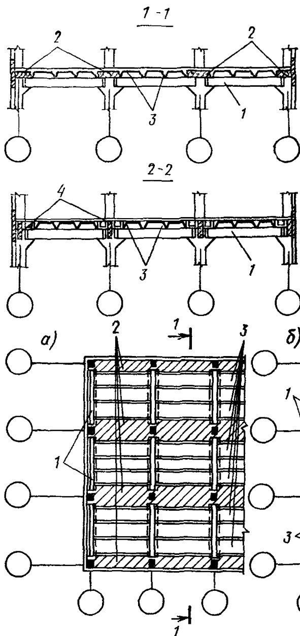
Рис. 48. Балочные перекрытия (покрытия) многоэтажного здания.
