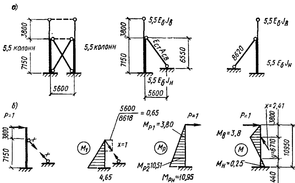
Рис. 108. Расчетная схема (а) и эпюры моментов от единичных сил (б) в колоннах здания по оси А и Б
