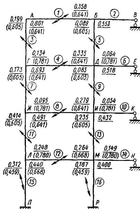
Рис. 116. Схема рамы с коэффициентами распределения и передачи
