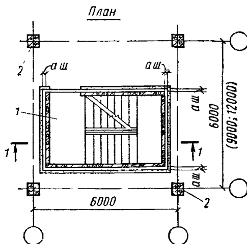
Рис. 93. Схема встроенной отдельно стоящей лестничной клетки
