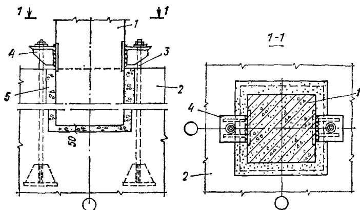
Рис. 68. Стык железобетонной колонны с фундаментом
