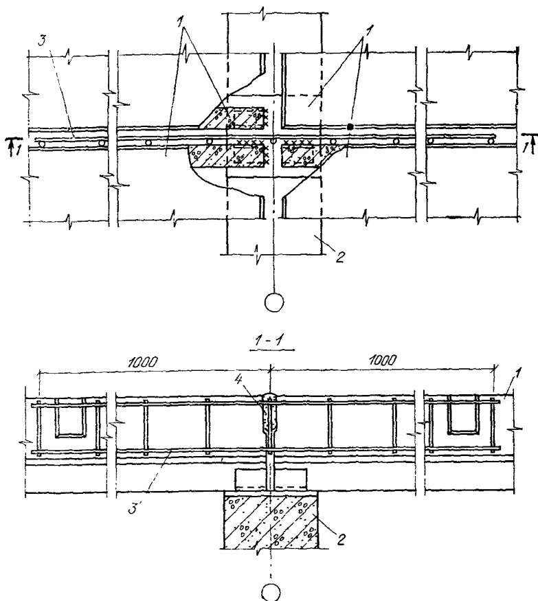
рис. 19. Установка каркаса между продольными ребрами плит покрытия 1 — плиты покрытия; 2 — стропильные конструкции; 3 — сварной каркас; 4 — цементный раствор марки 200
