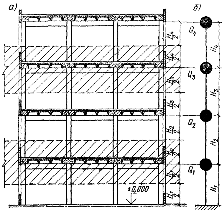
Рис. 49. Динамическая расчетная схема каркаса многоэтажного здания
