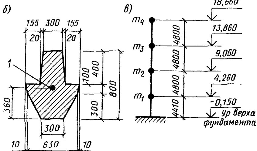
Рис. 112. Поперечный разрез здания (а), поперечное сечение ригеля (б), динамическая расчетная схема каркаса здания (в)
