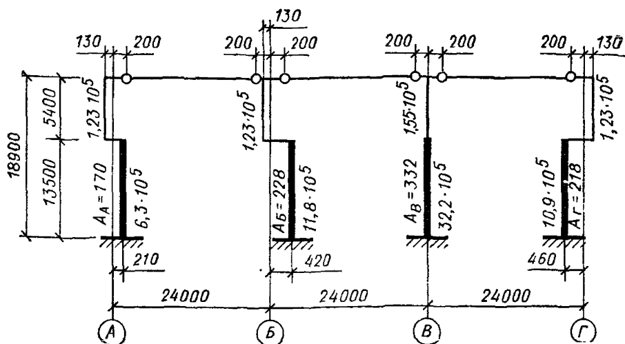
Рис. 132. Расчетная геометрическая схема поперечной рамы
