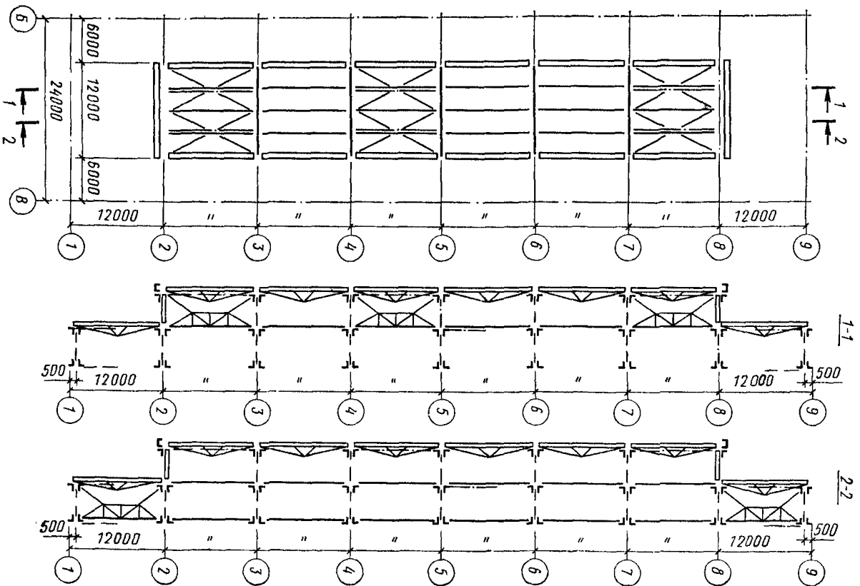
Рис. 142. План и разрезы по фронону
