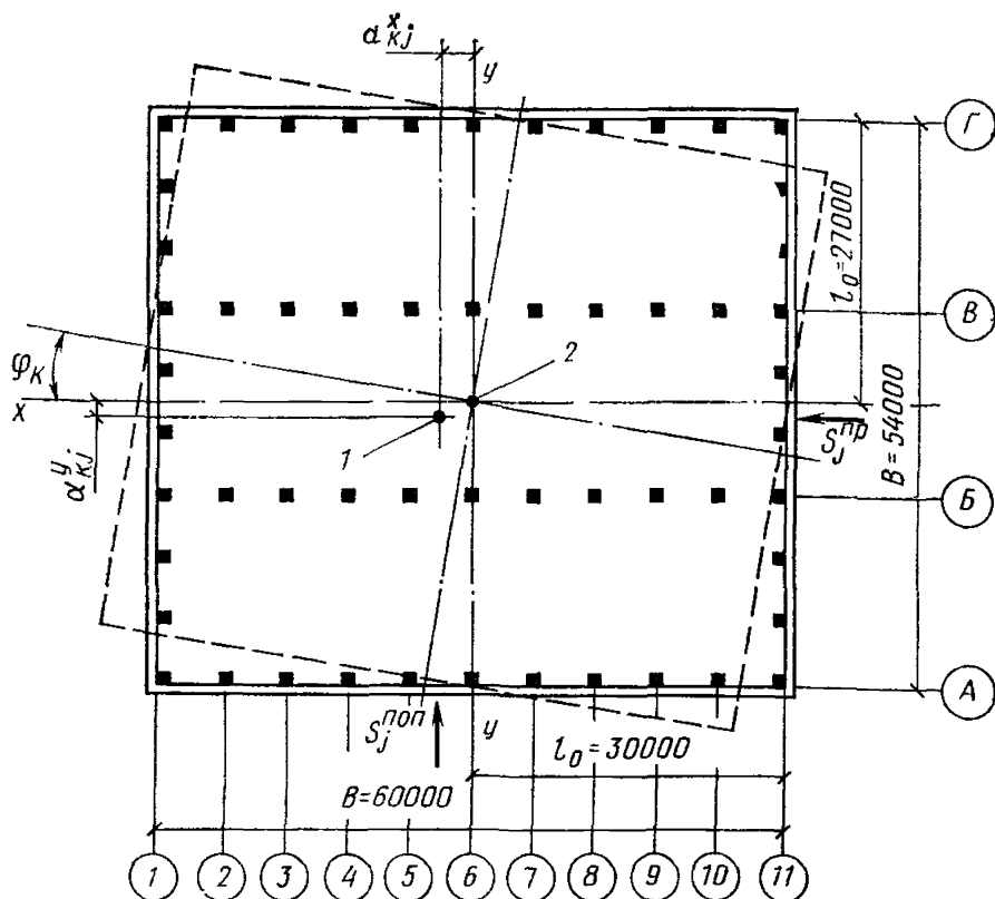
Рис. 99. Поворот здания в плане
