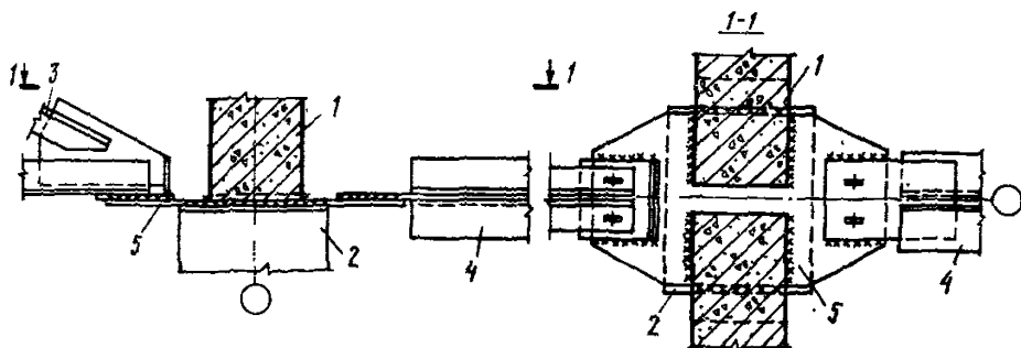
Рис. 26. Крепление вертикальной связи и распорки в покрытии здания с расчетной сейсмичностью 8 баллов в месте опирания стропильной фермы на колонну среднего ряда
