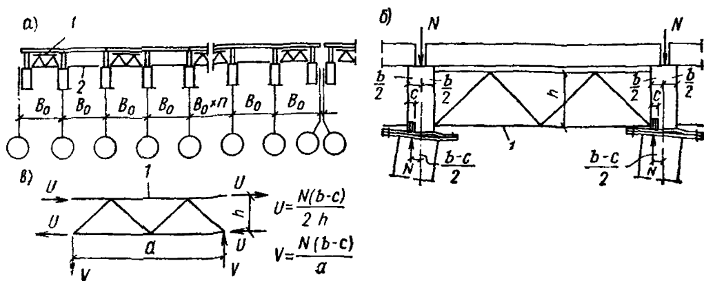
Рис. 32. Схемы к расчету вертикальных связей между опорными участками железобетонных стропильных конструкций на усилия от смещения места приложения вертикальной нагрузки на колонну
