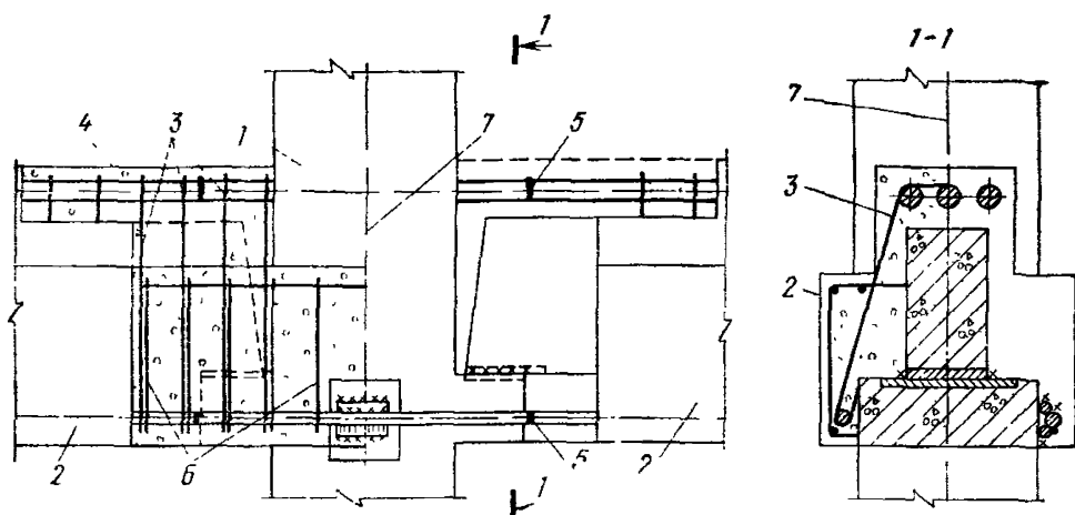
Рис. 52. Сопряжение сборных железобетонных ригелей с колонной
