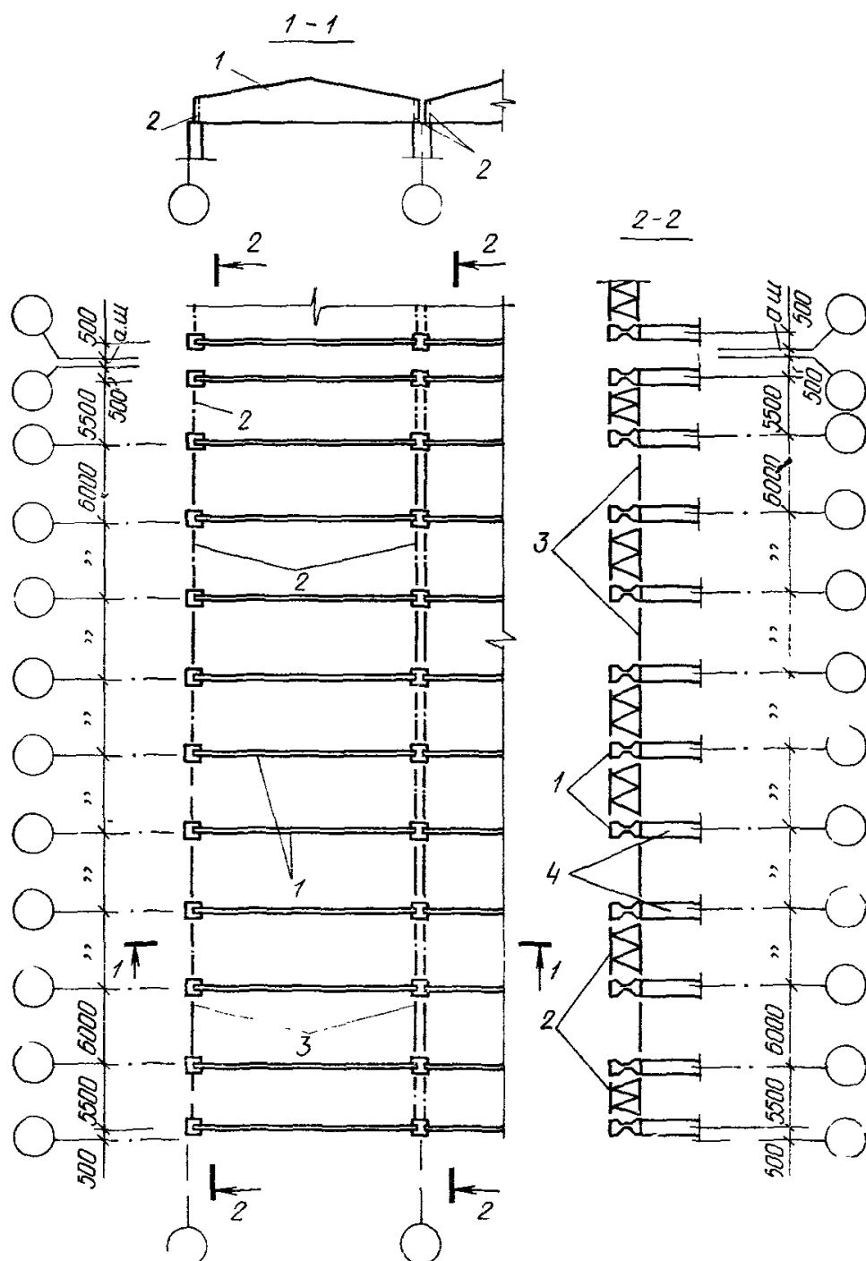
Рис. 30. Пример расположения связей покрытия с балками (при скатной кровле) в зданиях с расчетной сейсмичностью 9 баллов
