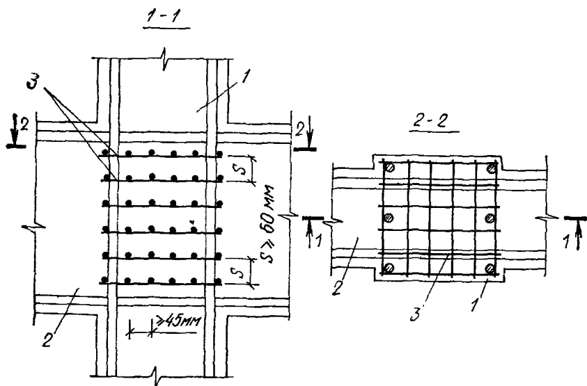
Рис. 58. Армирование центральной зоны узла сетками
