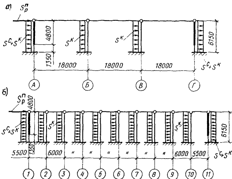
Рис. 100. Расчетные схемы рам каркаса
