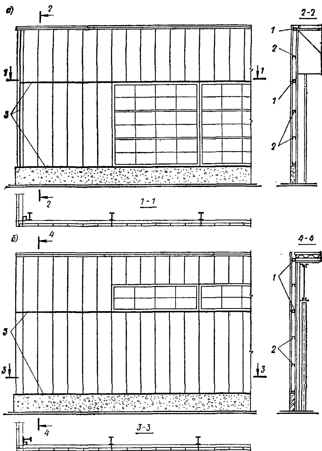
Рис. 74. Примеры решения металлических стен из трехслойных панелей
