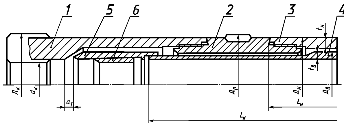
1 — коронка; 2 — расширитель; 3 — наружная колонковая труба; 4 — внутренняя керноприемная труба; 5 — корпус кернорвателя; 6 — керноприемное кольцо
