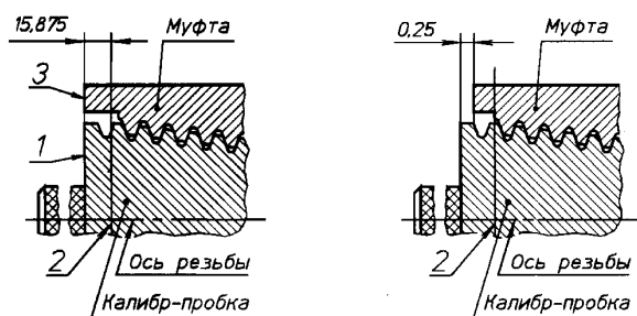
1 — контрольная плоскость; 2 — основная плоскость; 3 — упорный торец
