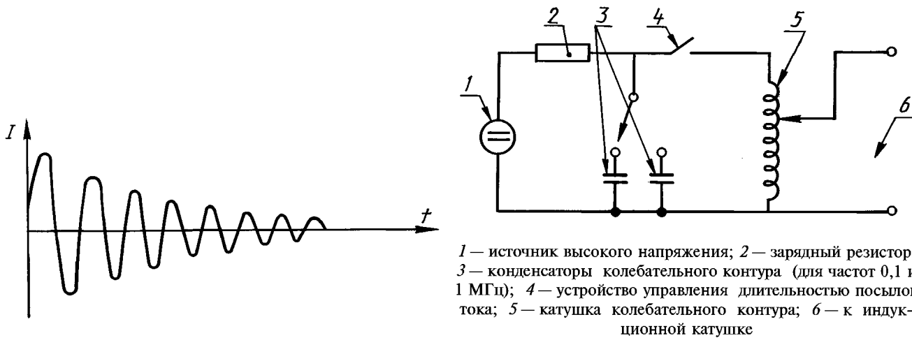
Рисунок 2 — Форма выходного тока ИГ
