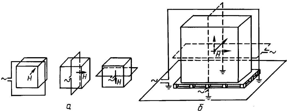
a — настольное ТС; б — напольное ТС
