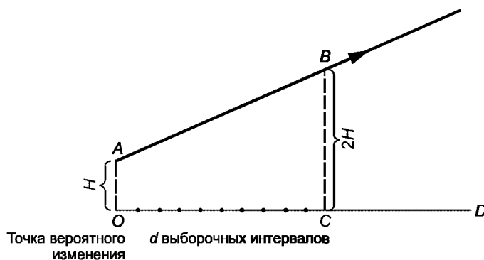
Рисунок Г.1 — Построение локальной разрешающей линии
