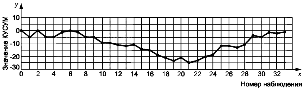
Рисунок В.1 — КУСУМ-карта для данных таблицы В.1 ( T = 15 )
