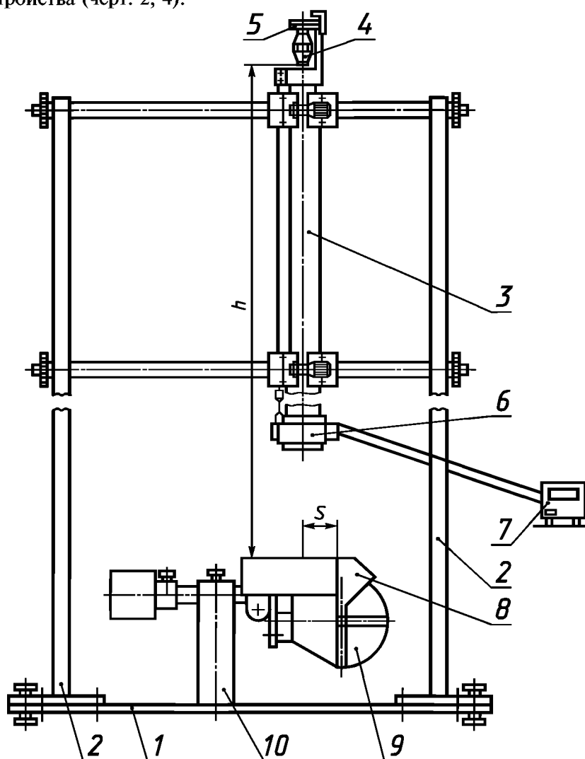
1 — станина; 2 — стойки; 3 — направляющая труба; 4 — ударник; 5 — спусковое устройство; 6, 7 — узлы счетчика времени; 8 — испытуемый щиток; 9 — макет головы человека по ГОСТ 12.4.128; 10 — устройство для закрепления щитка
