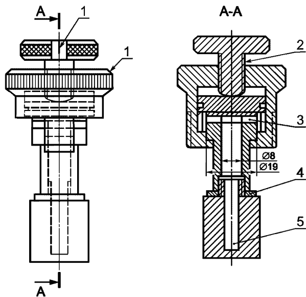
1 — вертикальная установочная метка; 2 — шаг 1 мм; 3 — проба; 4 — металлическая подкладочная шайба; 5 — внутренний объем 5,5 \text{ см}^3
