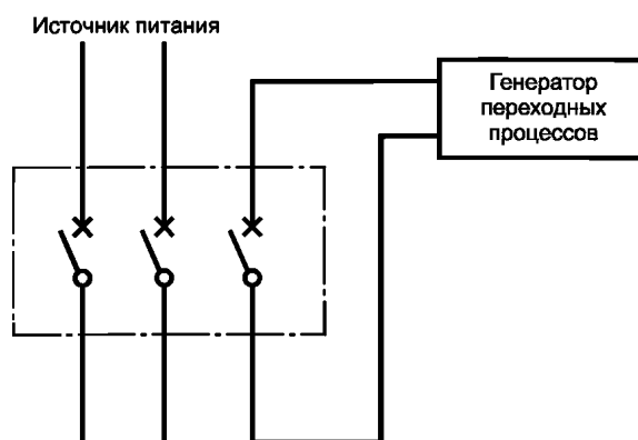
Рисунок F.4 — Испытательная цепь для проверки влияния электромагнитных помех в главной цепи (дифференциальный тип)
