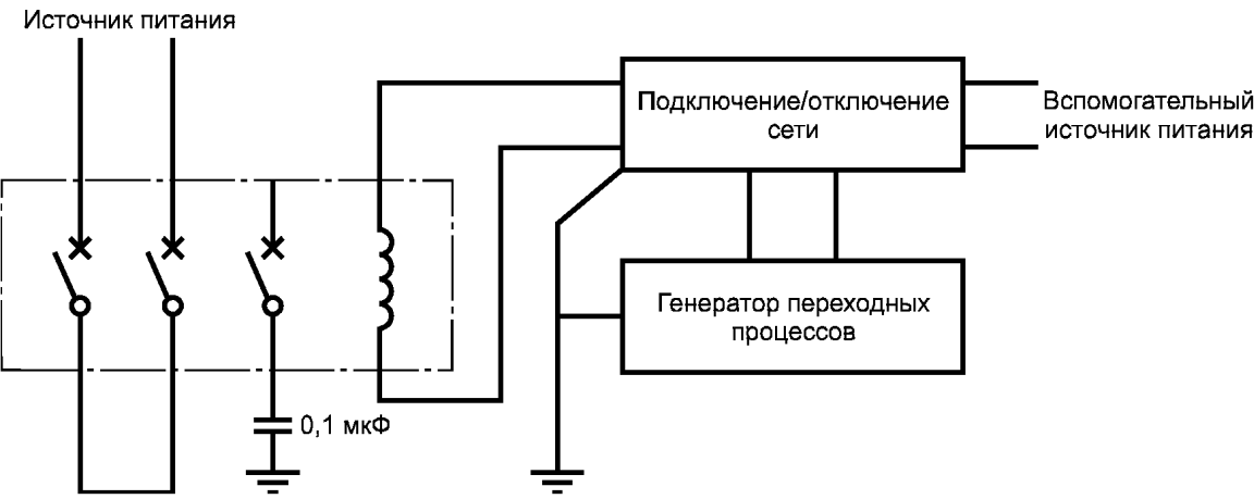
Рисунок F.6 — Испытательная цепь для проверки влияния электромагнитных помех во вспомогательных цепях (дифференциальный тип)
