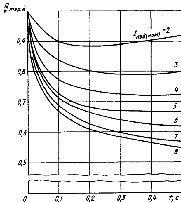
Кривые для определения Q_{*тер.д} от синхронного электродвигателя
