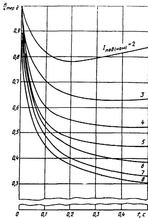
Кривые для определения B_{*тер.д} от синхронного электродвигателя
