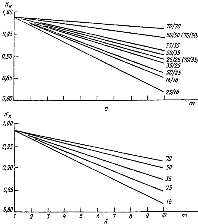
Поправочные коэффициенты ( K_R и K_X ) к активному и индуктивному сопротивлениям петли «фазовый провод — нулевой провод воздушной линии»
