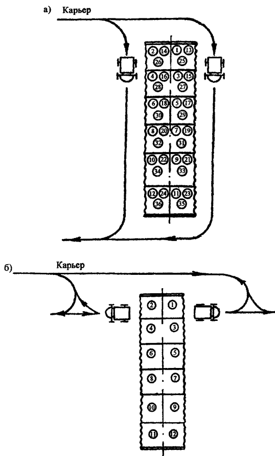
Рис. 9. Схемы движения автомобилей-самосвалов и уплотняющих механизмов при устройстве обоймы: а – при засыпке трубы в прогалах насыпи; б – при свободном подъезде; 1, 2 и т.д. – последовательность сторонности отсыпки
