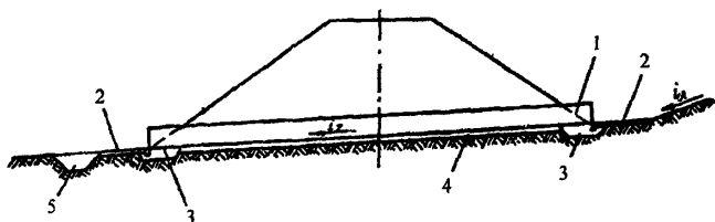
Рис. 2. Схема размещения трубы на косогоре: 1 – входной оголовок (без скоса); 2 – укрепление русла; 3 – противофильтрационный экран; 4 – подушка; 5 – отсыпка камней рисбермы
