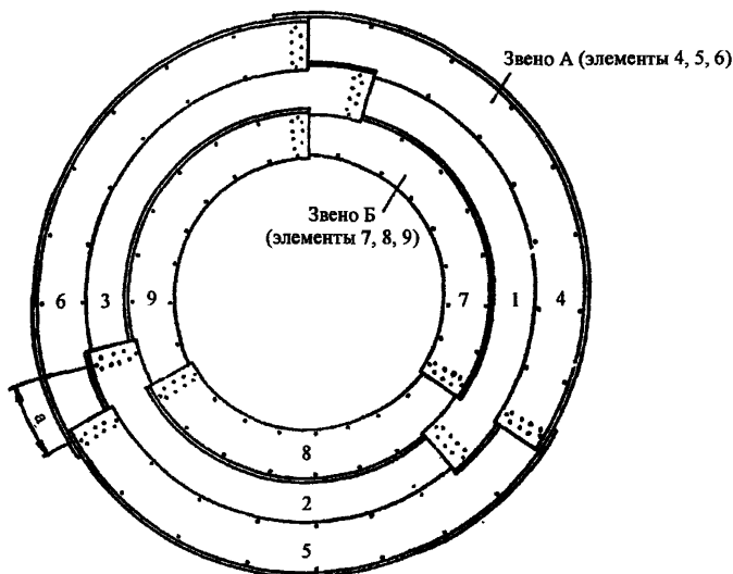
Рис. 5. Сборка секции трубы из звеньев ( d = 1,5 м, вид с торца): цифрами показан порядок установки элементов; а – сдвигка (забег) продольных стыков
