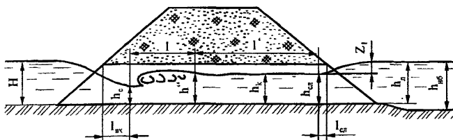
Рис. 3. Схема протекания воды в безнапорной трубе, подтопленной с нижнего бьефа, с незатопленным сжатым сечением
