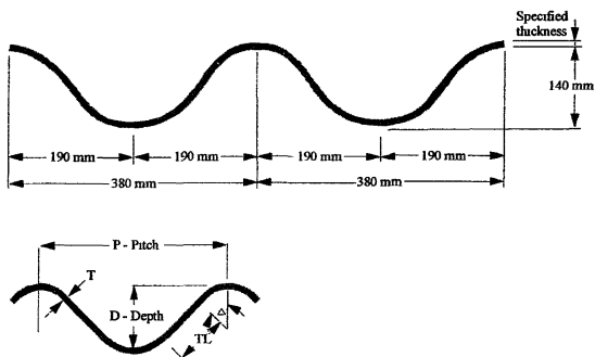
Рис. 3. Профиль гофрированного листа: толщина листа 2,75-7,0 мм
