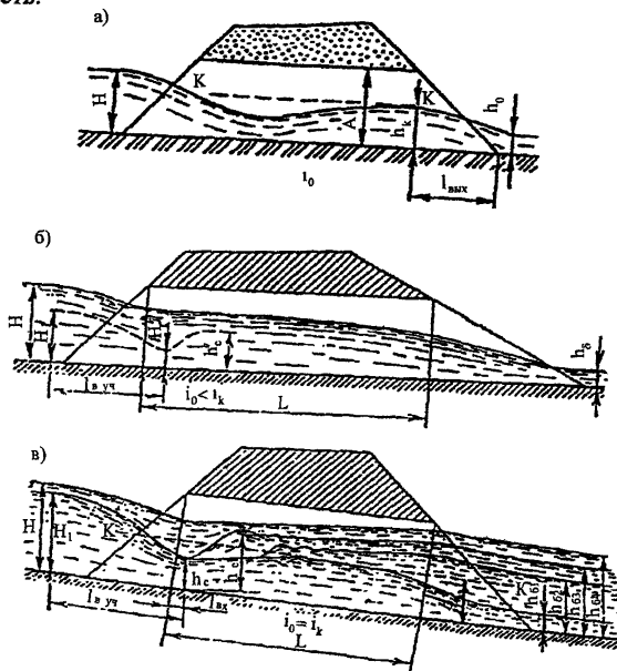
Рис. 1. Схема протекания воды в равнинной трубе при безнапорном режиме: а – «короткая»; б – «длинная»; в – «незатопленная» ( h_{62}, h_{63} ) и «затопленная» с нижнего бьефа ( h_{64} )
