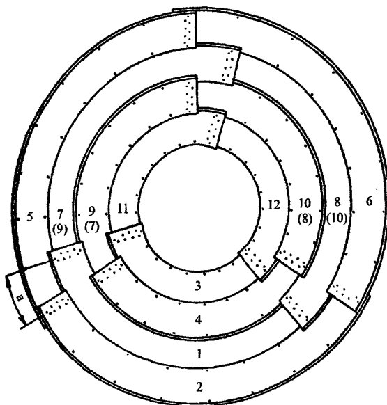
Рис.8. Сборка труб из элементов на оси сооружения ( d = 1,5 м, вид с торца): цифрами показан порядок установки элементов; a – сдвигка (забег) продольных стыков
