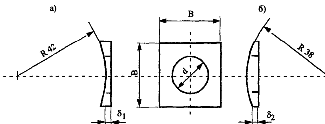
Рис. 1. Шайбы для болтов (размеры в мм): а — плоскогогнутые; б — плосковыпуклые; d — диаметр отверстия в шайбе (согласно ГОСТ 11371-68*); B — размер квадратной шайбы, принимаемый равным наружному диаметру стандартной круглой шайбы (согласно ГОСТ 11371-78*); \delta_1 — не менее 3; \delta_2 — не менее 2
