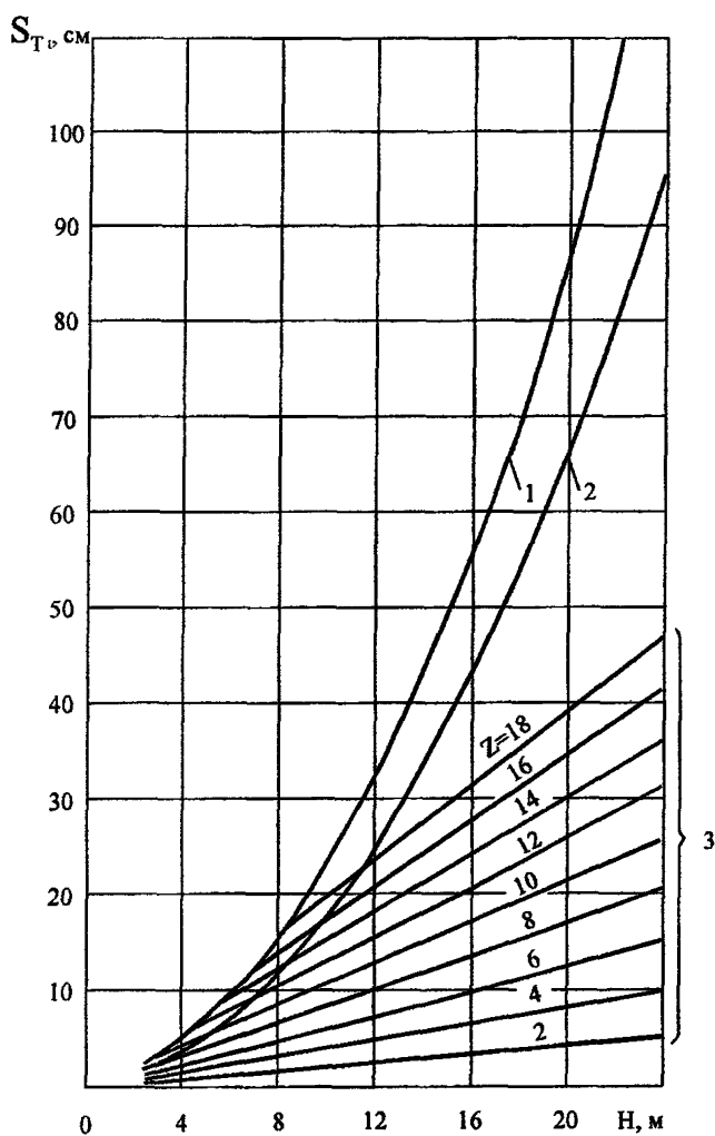
Рис. 1. Расчетный график для определения осадки трубы: S_T – осадка основания при модуле деформации грунта 100 \text{ кг/см}^2 ; H – высота насыпи; Z – расстояние от нижней границы слоя до верха основания; 1, 2 – при однородном основании и \gamma = 1-1,7 \text{ т/м}^3 ; 3 – при неоднородном основании
