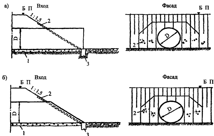
Рис. 1. Схема конструкции трубы верховой стороны насыпи: 1 – подушка основания; 2 – укрепление откоса; 3 – противодиффузионный экран
