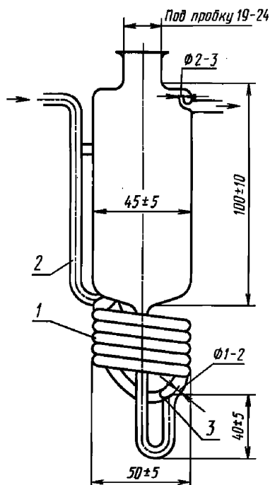
1 — пять полных витков трубки диаметром (6±1) мм; 2 — стеклянная перемычка; 3 — место впаива газопроводящей линии
