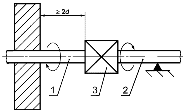
d — наружный диаметр 1, 2 — труба; 3 — испытываемый образец
