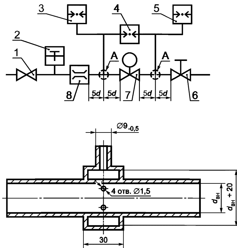
A — деталь; d_{\text{вн}} — внутренний диаметр трубы; d — наружный диаметр трубы 1 — регулятор давления; 2 — термометр; 3, 5 — манометры; 4 — дифференциальный манометр; 6 — регулировочный кран; 7 — испытуемый образец; 8 — расходомер
