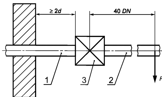
d — наружный диаметр трубы 1, 2 — труба; 3 — испытуемый образец
