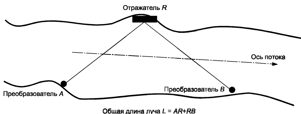
Рисунок 2 — Схема расположения преобразователей с отражением лучей
