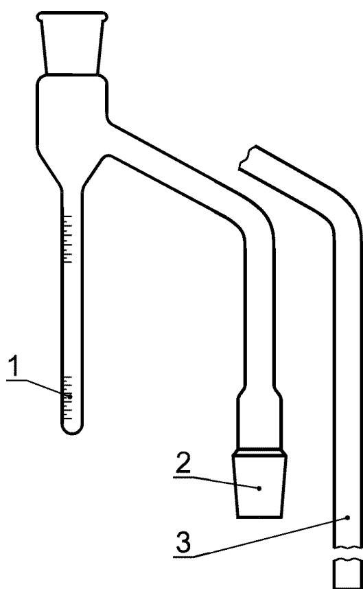
1 — градуировка ценой деления 0,05 \text{ см}^3 ; 2 — керн; 3 — простое соединение
