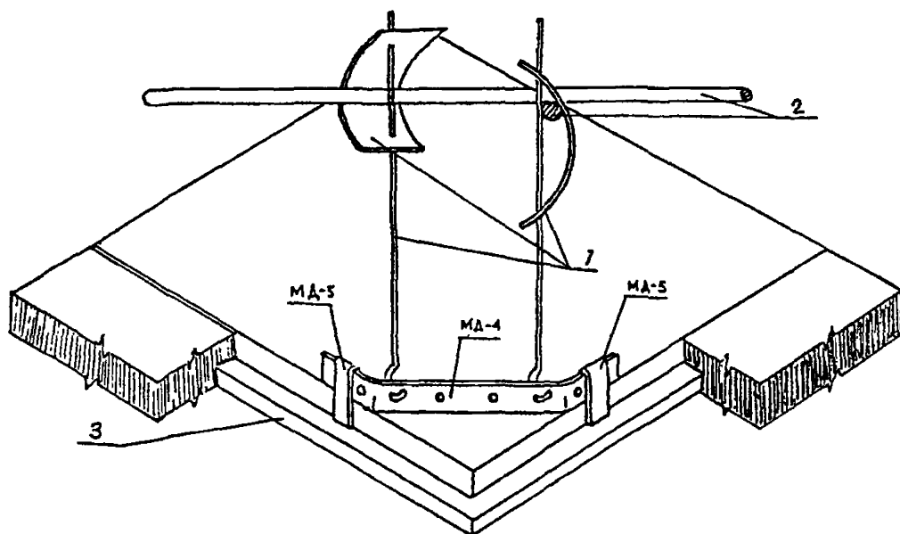
Р и с. 7. Подвесной потолок из гипсовых декоративных плит "ГРП": 1 — подвеска ПП-2; 2 — несущая арматура; 3 — гипсовая декоративная плита
