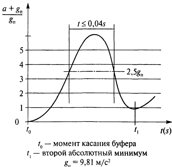
Рис. 1. График торможения
