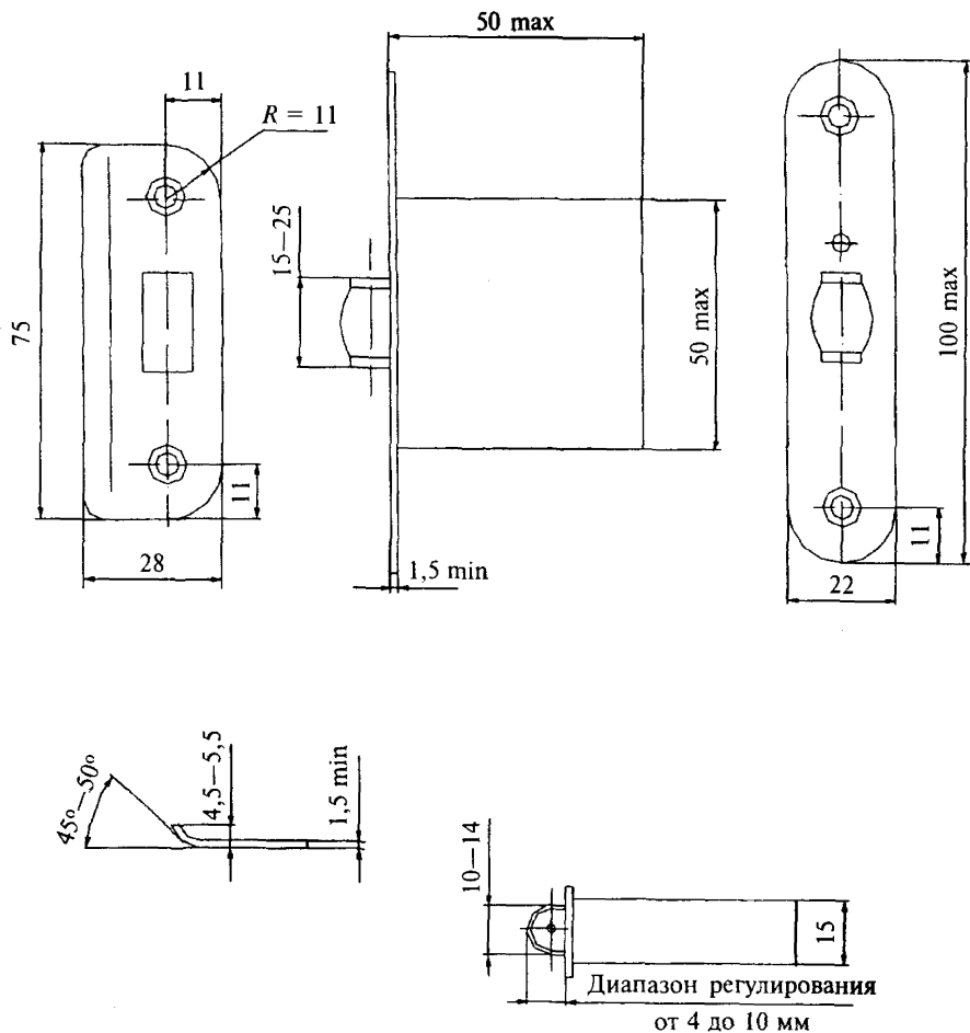
Рисунок В.22 — Пример защелки врезной типа ЗЩ4
