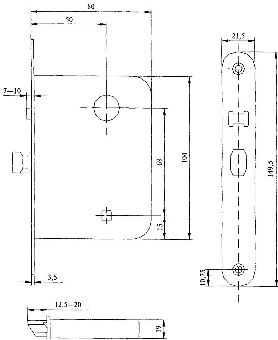
Рисунок В.9 — Пример замка врезного цилиндрического типа ЗВ7 с автоматическим выводом засова-зашелки
