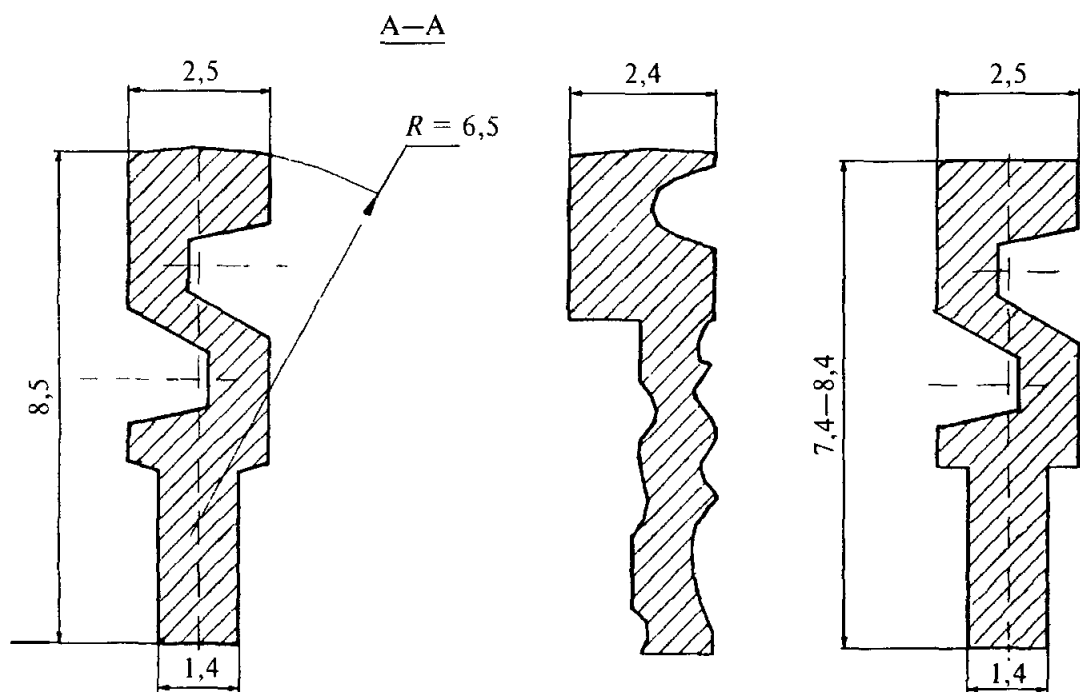
Варианты профиля ключа
