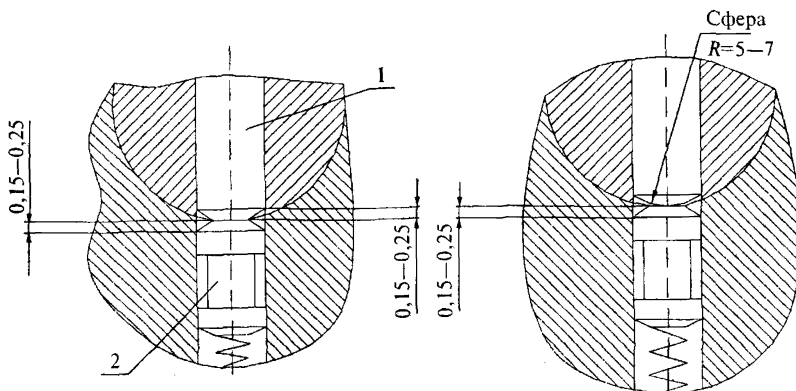
1 — штифт цилиндра; 2 — штифт корпуса
