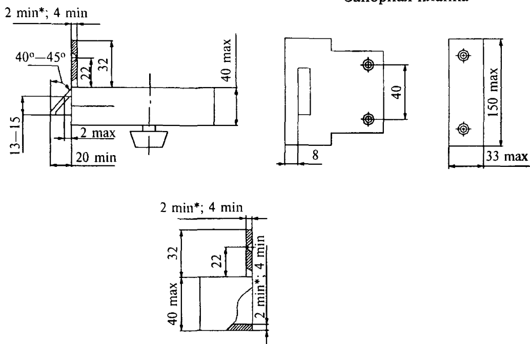
Запорная планка
