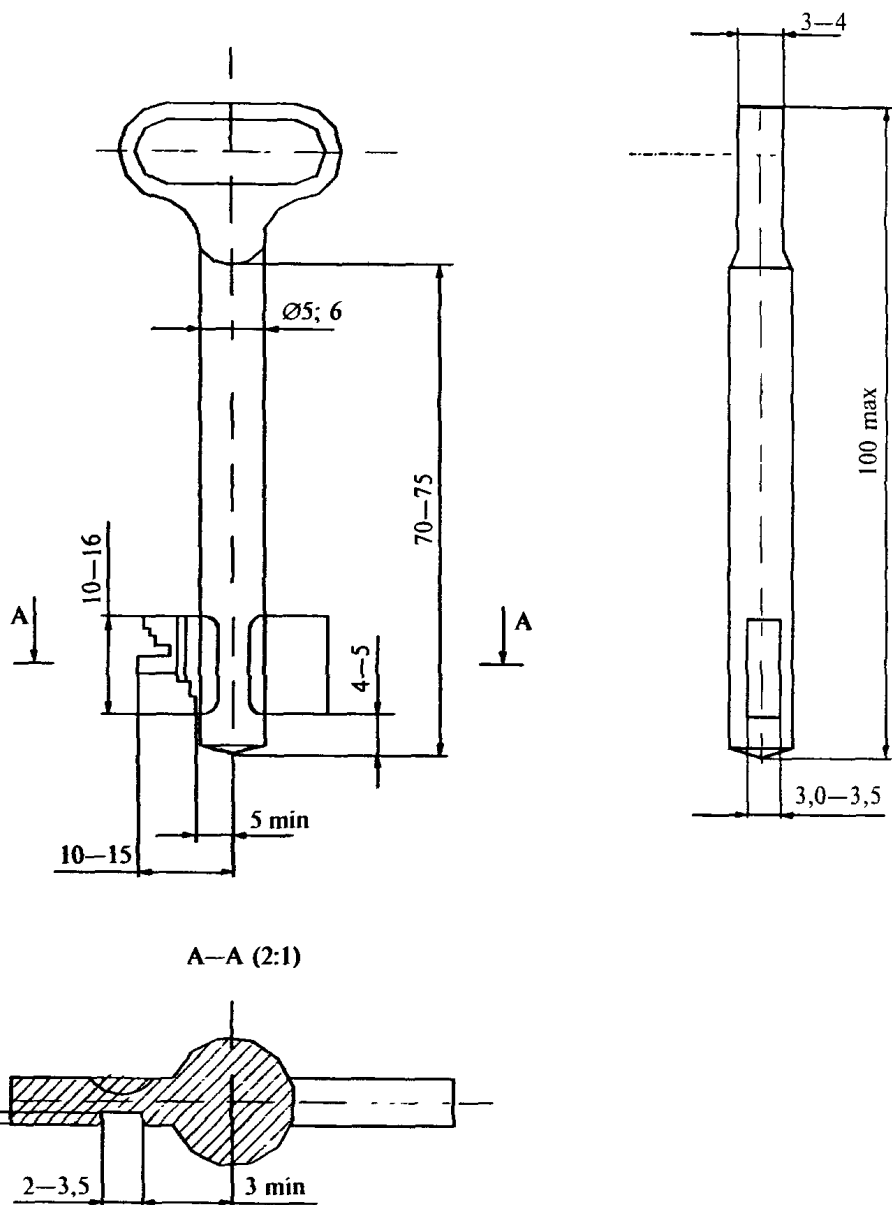
Рисунок В.47 — Пример ключа для накладного сувальдного замка, тип 3С2
