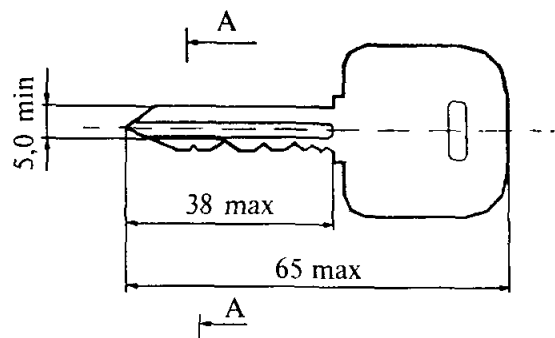
Варианты профиля ключа
