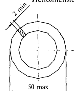
Рисунок В.42 — Примеры накладок для цилиндрических и сувальдных замков, тип Н4
