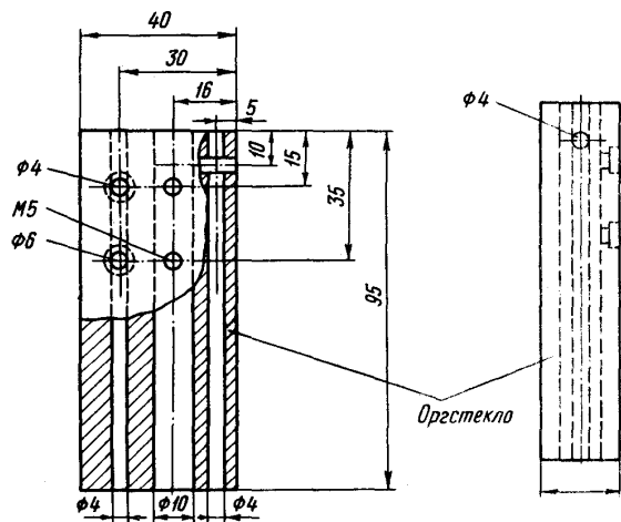
Рис.5. Верхняя часть реометра
