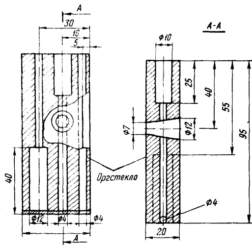
Рис.6. Нижняя часть реометра
