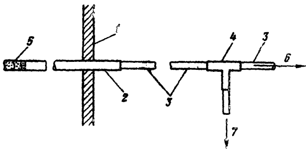
Рис.2. Схема отбора пробы газа для анализа прибором "Радиометр-2": 1 - стенка газохода; 2 - пробоотборник; 3 - соединительный шланг; 4 - тройник; 5 - фильтр (анализируемый газ); 6 - к эжектору; 7 - к прибору
