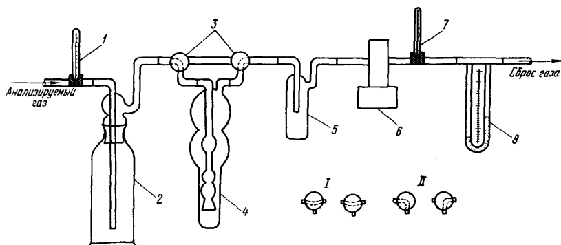
Рис. I. Принципиальная схема прибора "Эвдиометр-2":
