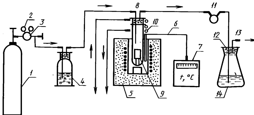
Схема установки для определения азота в карбидкремниевых огнеупорах на связках из нитрида и оксинитрида кремния
