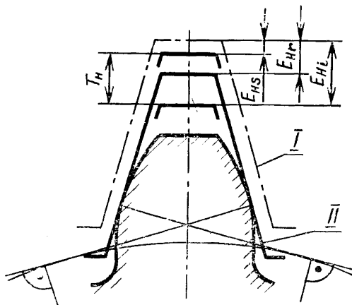
I—номинальное положение исходного контура; II—действительное положение исходного контура.
