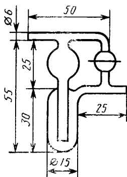
Склянка Дрекслея с краном
