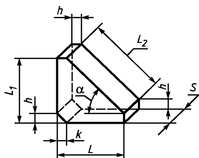
Рисунок 7 — Кирпич пятовый
