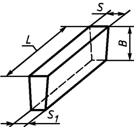
Рисунок 3 — Клин ребровый двухсторонний
