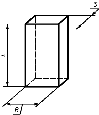
Рисунок 1 — Кирпич прямой
