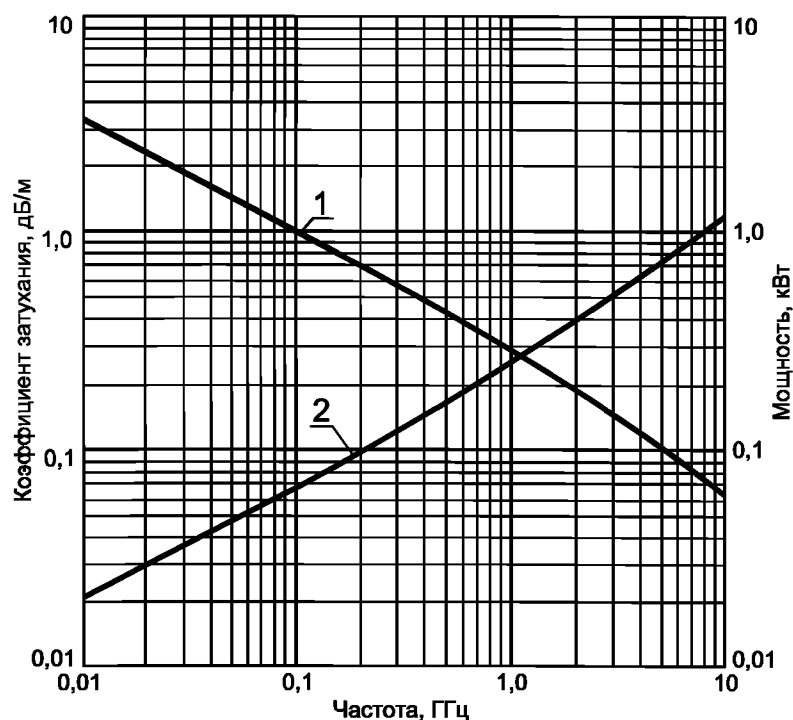
Частотные зависимости
