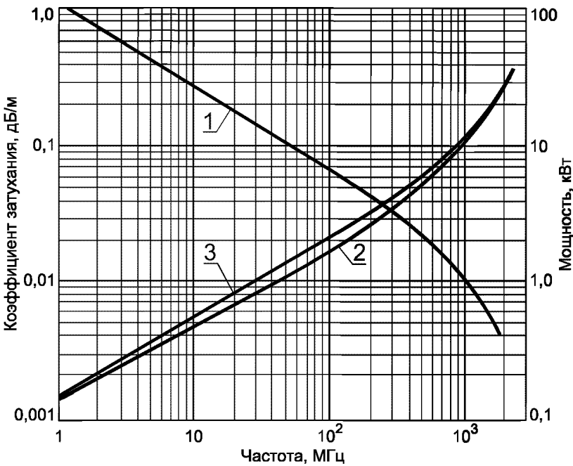
Частотные зависимости
