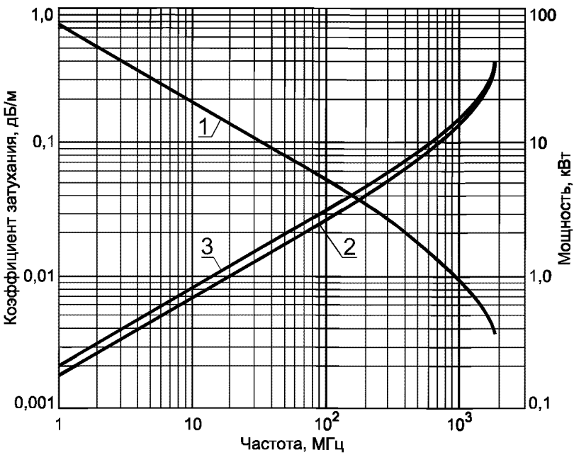
Частотные зависимости
