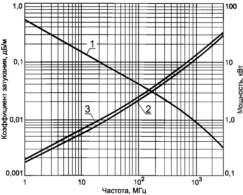
Частотные зависимости
