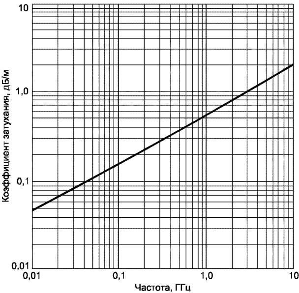
Частотная зависимость коэффициента затухания \alpha при температуре 20 °С
