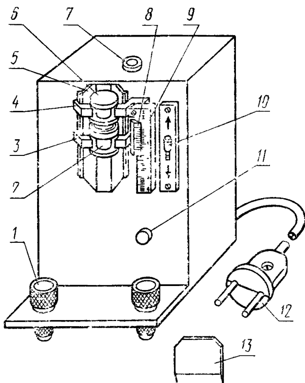
1—маховичок; 2—кювета; 3—каретка. 4—установочная планка; 5—экран, 6—конус; 7—уровень; 8—нониус; 9—шкала; 10—рукоятка ключа; 11—предохранитель; 12—штепсельная вилка; 13—шпатель.
