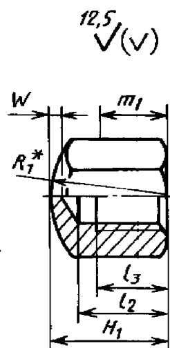
Исполнение 2
