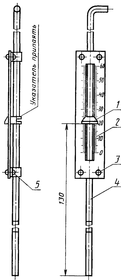
1—указатель; 2—шкала; 3—заклепка; 4—игла; 5—скоба
