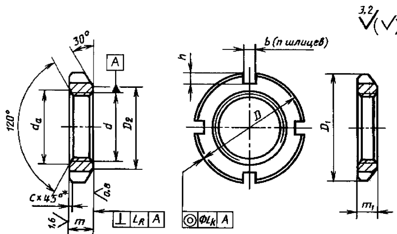
Исполнение 1
