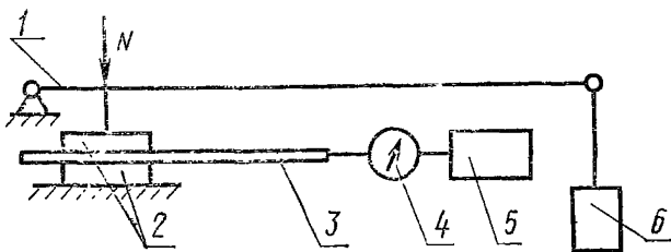
1—нажимной рычаг; 2—образец; 3—стальная испытательная полоса; 4—измерительный прибор; 5—привод; 6—груз
