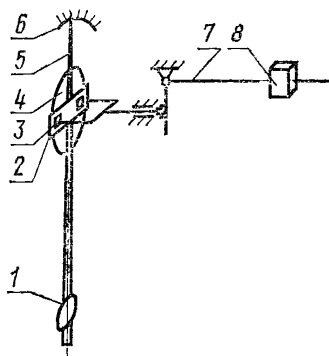
1—маятник; 2—держатель образцов; 3—образец; 4—кольцо чугунное; 5— стрелка-указатель; 6—шкала; 7—ры- чажная система; 8—груз
